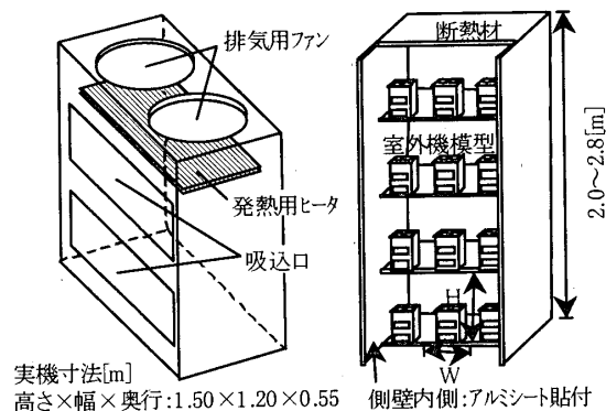
図1 室外機模型
