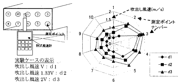
図4 室外機吹出し風速比較
