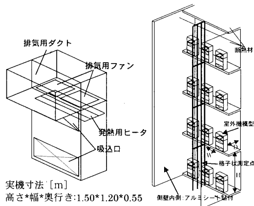
図1 室外機模型
