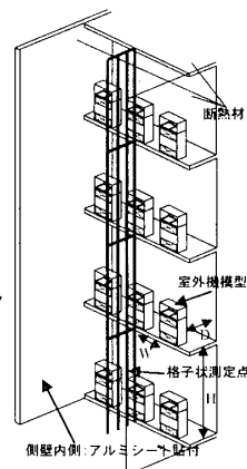
図2 装置配置
