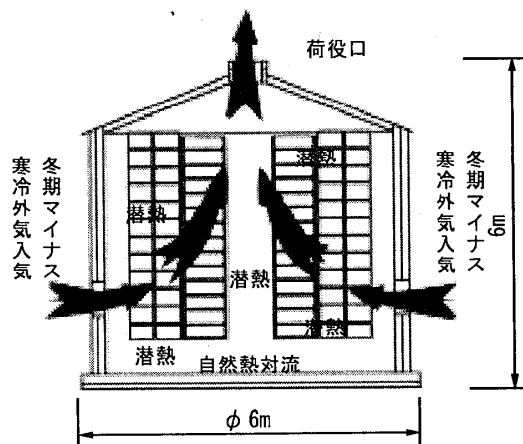
図1 アイスシェルターの製氷原理図
