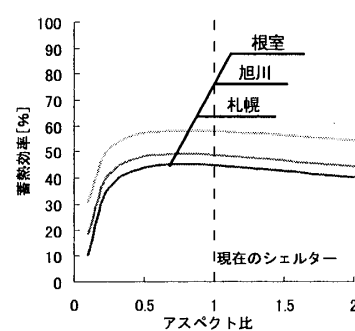
図6 アスペクト比の検討
