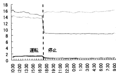
図3 アイスシェルター内垂直温度分布
