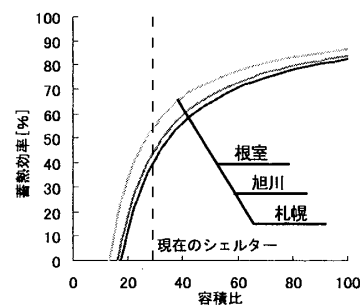
図7 容積比と蓄熱効率の関係
