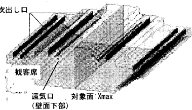
図3 CFD解析対象モデル
