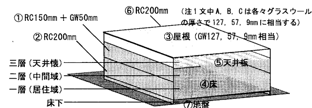
解析対象モデル
