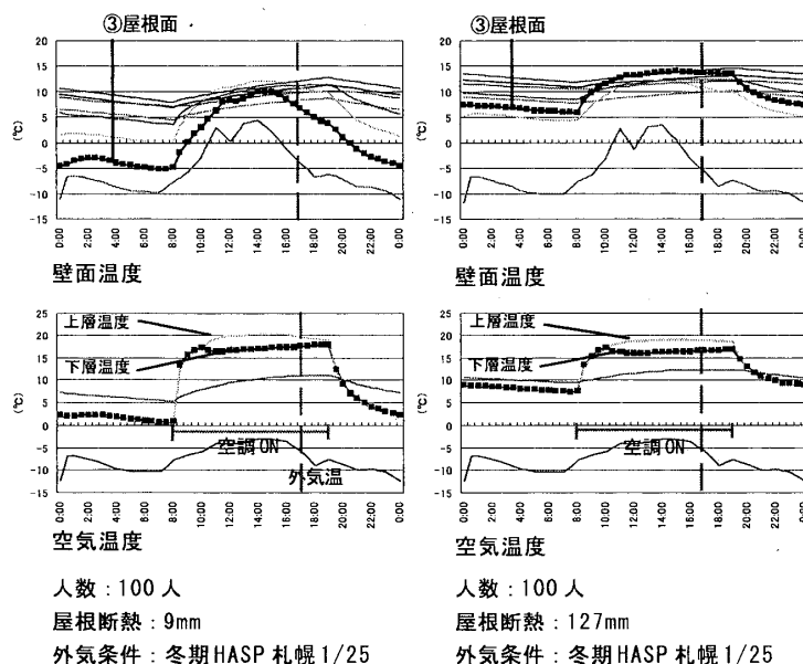
図2 ブロックモデル解析結果
