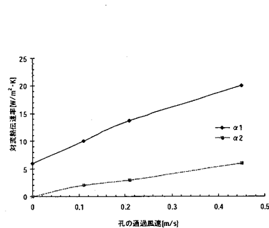
図9 孔の通過風速と対流熱伝達率の関係
