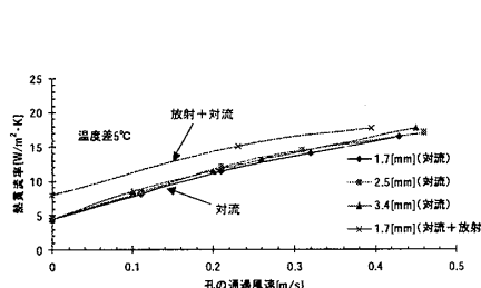
図7 孔径をパラメータとした場合の孔の通過風速と熱貫流率の関係
