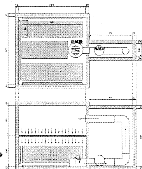
図5 実験装置の平面図と断面図
