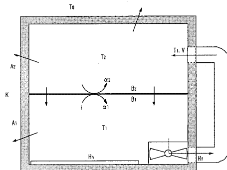
図8 熱移動のモデル化
