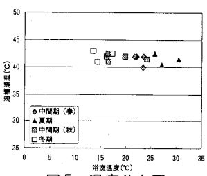
図5 温度分布図 (札幌・住宅②)
