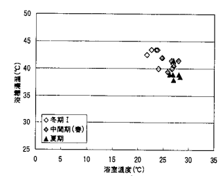
図6 温度分布図 (旭川・住宅⑥)
