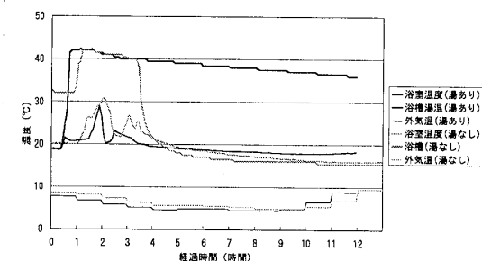
図7 浴室まわりの温熱環境の時系列変化(札幌・住宅②)
