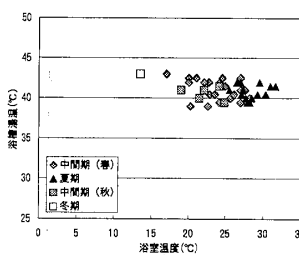
図3 温度分布図 (札幌・0～39歳)
