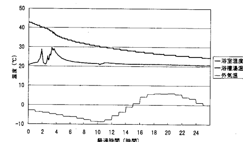
図8 浴室まわりの温熱環境の時系列変化(旭川・住宅⑥)
