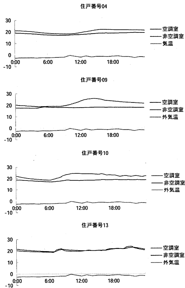
図1 各住宅における室内外温度(2004年1月25日)
