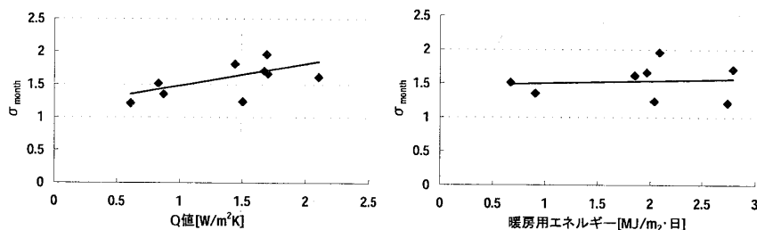
図4 熱損失係数および暖房用エネルギーと室温標準偏差
