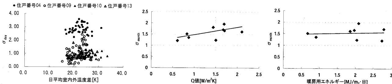
図3 室内外温度差と室温標準偏差
