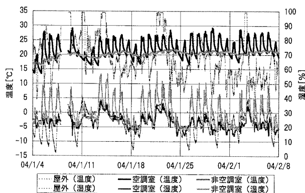
図3 空調室と非空調室の温湿度変動
