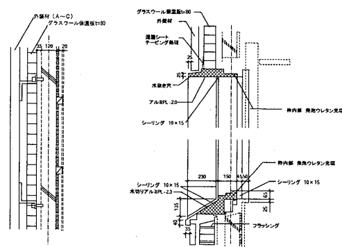
図1 改修後の壁・窓断面詳細
