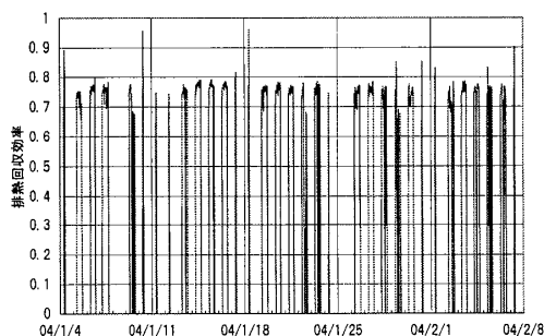
図5 排熱回収効率の推移
