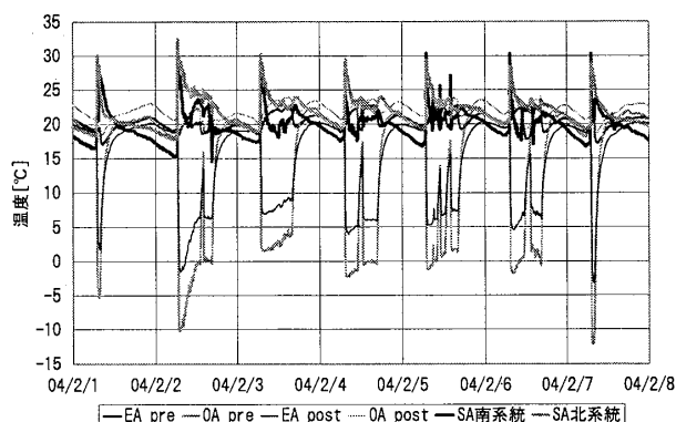
図4 全熱交換器・空調機まわり空気温度変動
