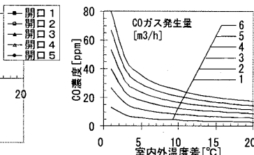
図 9 CO ガス濃度
