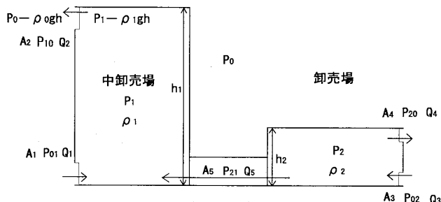
図 7 換気モデルの概要
