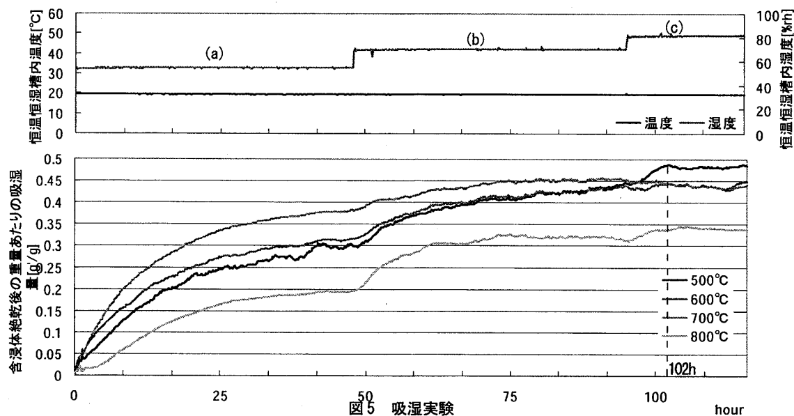
図5 吸湿実験
