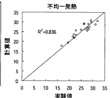
図 6 吸込み温度の整合性
