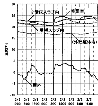
図5 スラブ内の温度変動
