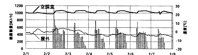
図6 熱源熱量と室温変動
