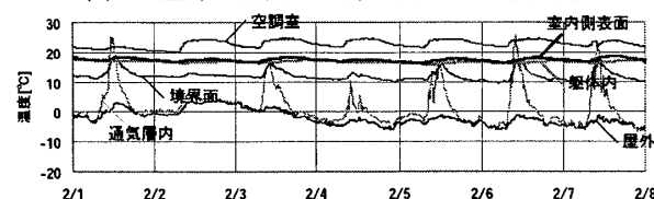
図4 外壁躯体の温度変動
