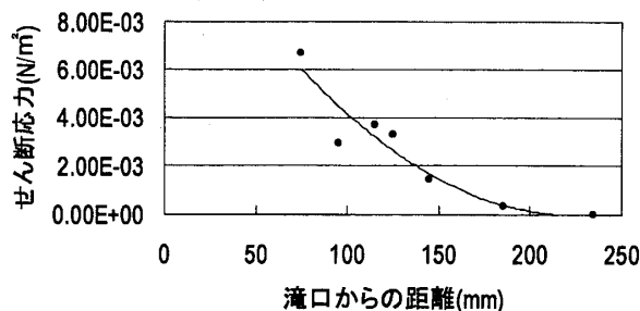
図-7 境界面に働くせん断力(流量12.2 l/min)
