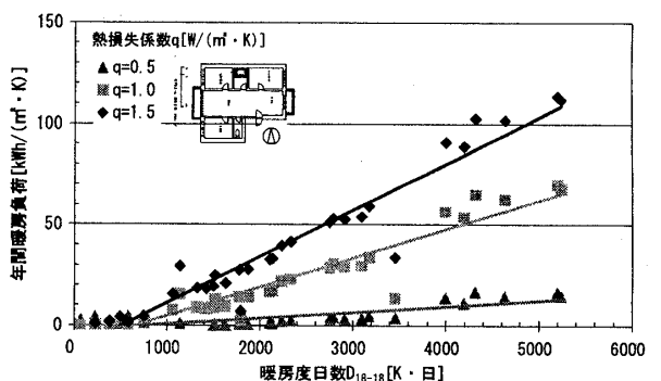
図6 各都市の年間暖房負荷(東西面開口)
