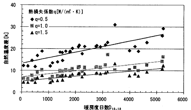
図4 各都市の自然温度差
