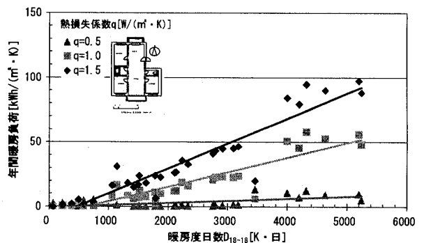
図5 各都市の年間暖房負荷(南北面開口)
