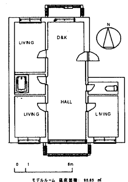
図 2 住戸の平面図
