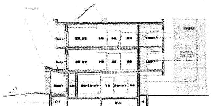
図4 換気計画
