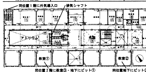
図 2 3階平面図
