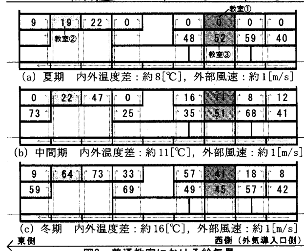
図2 普通教室における給気量
