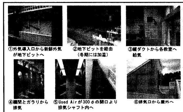
図1 換気経路
