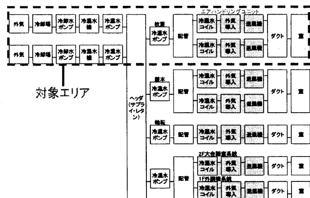
図 2 対象建物空調システム
