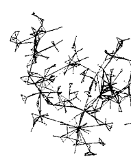
図 2: DSSOM
