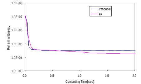
図6 ポテンシャルエネルギーの変化 Fig.6 Potential Energy (College football)
