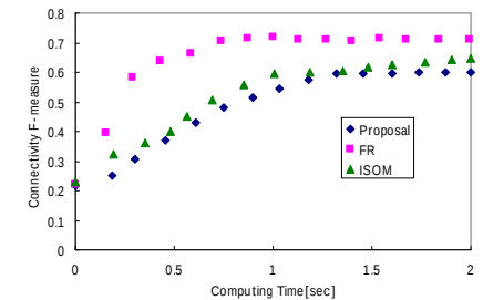
図8 College football における接続 F 尺度の変化 Fig.8 F-measure (College football)
