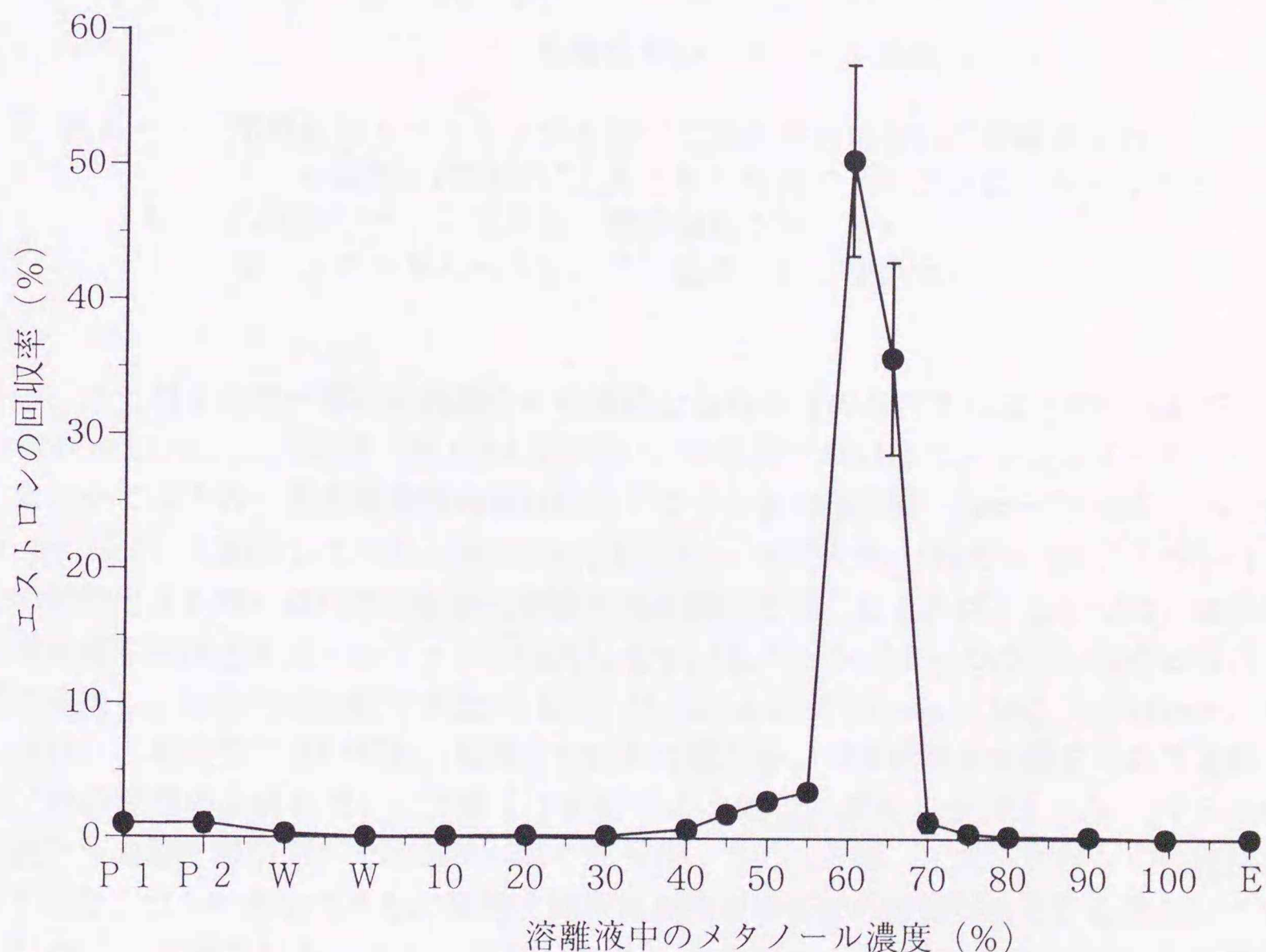
図2-1. 簡易逆相カートリッジを用いた固相抽出において溶離液中のメタノール濃度を段階的に上昇させた時のエストロンの溶出パターン (平均±標準偏差; N=5)
