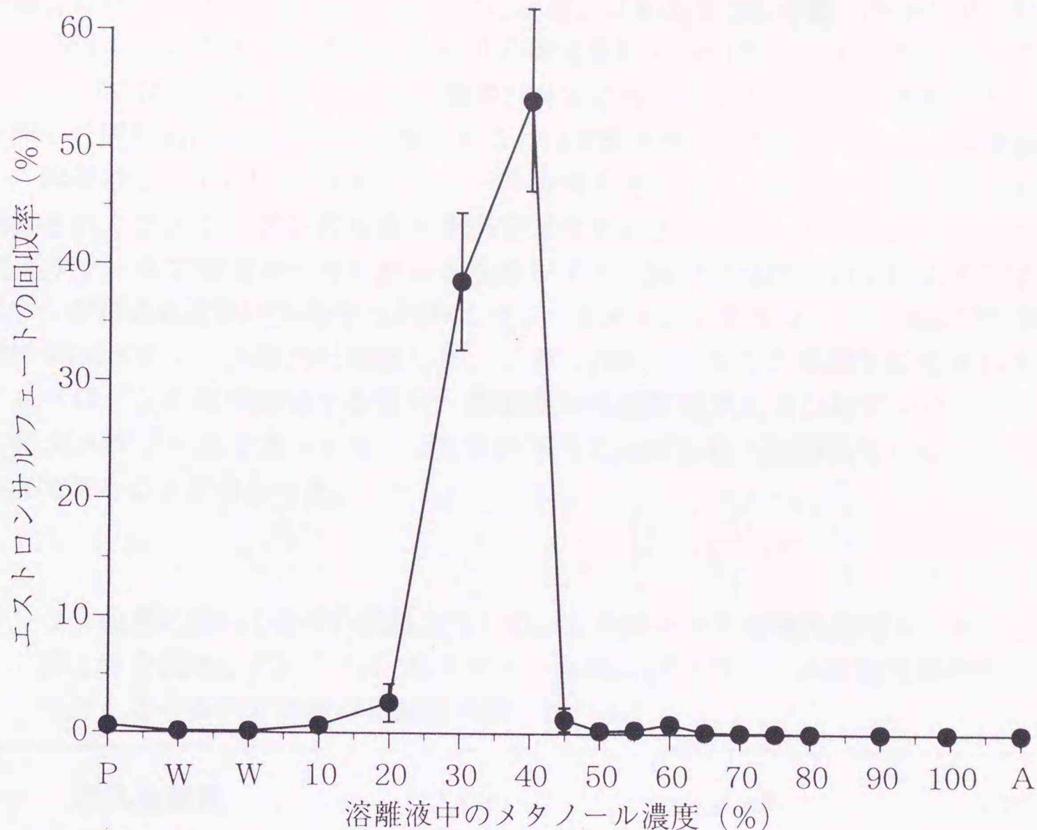
図2-3. 簡易逆相カートリッジを用いた固相抽出において溶離液中のメタノール濃度を段階的に上昇させた時のエストロンサルフェートの溶出パターン (平均±標準偏差; N=8 \times 2 ) A: アセトン、P: 血漿、W: 洗浄水
