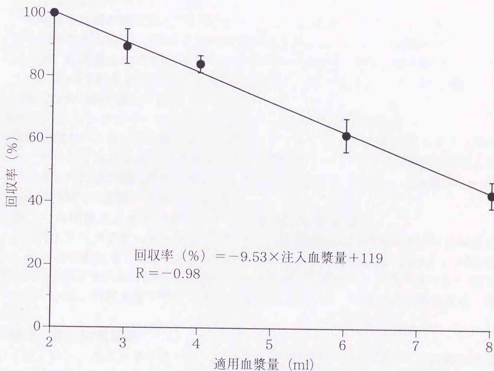
図3. 固相抽出物から直接RIAでエストラジオール-17 \beta を測定した場合に 注入量2 mlで測定した濃度を100%とした時の注入血漿量と濃度との 関係 (平均 \pm 標準偏差; N=5)
