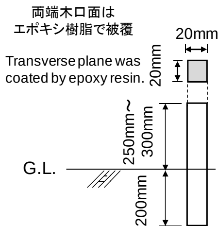
図 1. 試験体寸法
