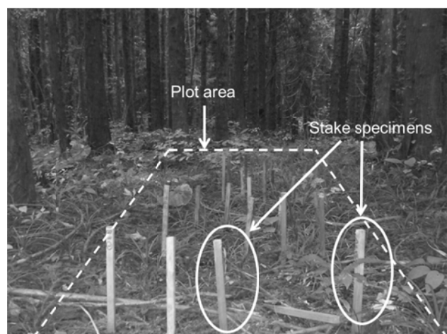
写真 1. 試験地概観
