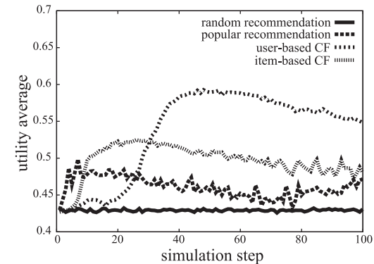
図 2 推薦アルゴリズムによる効用の平均値の推移 ( \mathbf{p}_i は一様分布, N_{\text{user}} = 500 , N_{\text{item}} = 500 )
