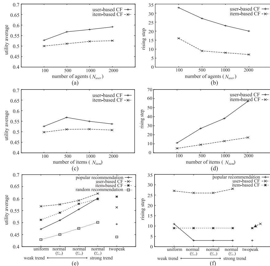
図3 各推薦アルゴリズムにおける、のピーク値および立ち上がりステップ。ただし、(a), (b) は, N_{item} = 500 , \mathbf{p}_i を一様分布として固定し, N_{user} = \{100, 500, 1000, 2000\} での実験結果。(c), (d) は, N_{user} = 500 , \mathbf{p}_i を一様分布として固定し, N_{item} = \{100, 500, 1000, 2000\} での実験結果。(e), (f) は, N_{user} = 500 , N_{item} = 500 で固定し \mathbf{p}_i の分布を変化させたときの実験結果
