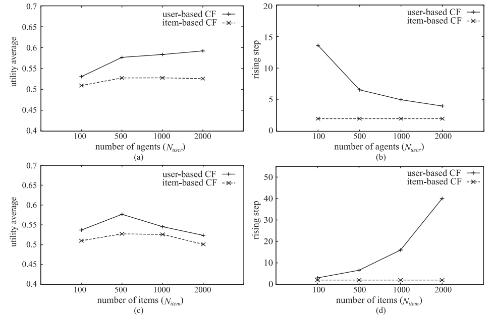
図 5 推薦システムにあらかじめ格付けが入力された状態における新規エージェントに対しての効用のピーク値および立ち上がりステップ。ただし、(a), (b) は N_{\text{item}} = 500 , \mathbf{p}_i を一様分布として固定し、 N_{\text{user}} = \{100, 500, 1000, 2000\} での実験結果。(c), (d) は N_{\text{user}} = 500 , \mathbf{p}_i を一様分布として固定し、 N_{\text{item}} = \{100, 500, 1000, 2000\} での実験結果
