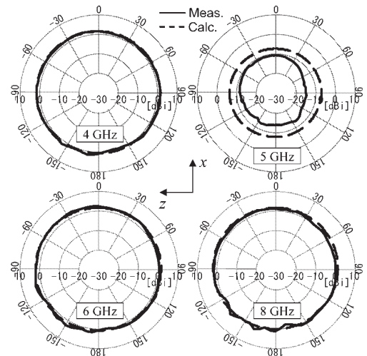
図 9 xz 面での放射パターン測定・解析結果
