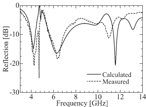
図 7 反射係数の解析・測定結果
