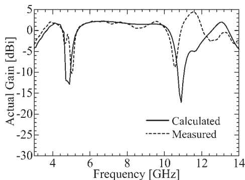
図 8 動作利得の解析・測定結果
