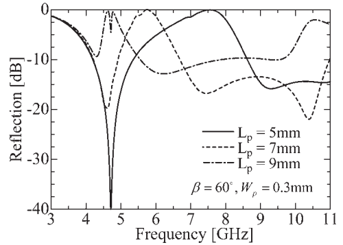
図 2 ストリップ導体長に対する反射係数の変化
