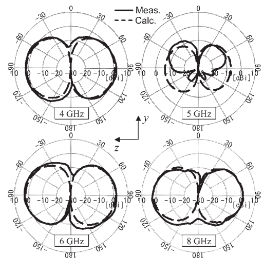
図 10 yz 面での放射パターン測定・解析結果
