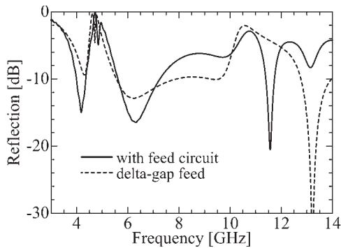
図 6 給電回路接続時とデルタギャップ給電時の反射係数の解析結果
