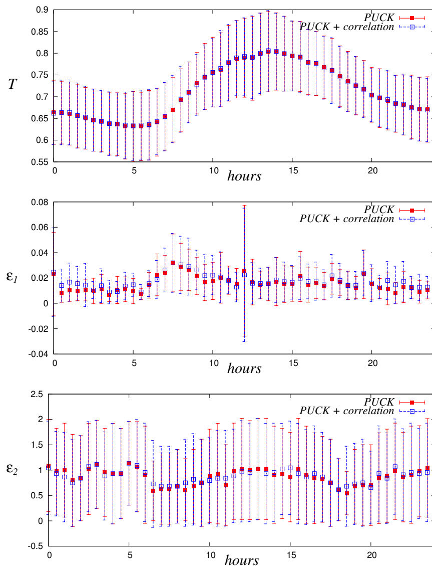
図 5: 上から札幌市気温の予測曲線, 誤差 \varepsilon_1^{(T)}, \varepsilon_2^{(T)} の時刻依存性. 誤差棒は 23 日分のデータから算出された標準偏差.
