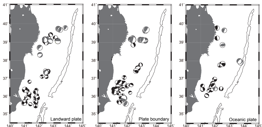
Fig. 4. 海底地震計で記録された P 波初動極性から決定された震源メカニズム解. 発生場所によって余震を上盤の陸側プレート内, プレート境界, 太平洋プレート内の地震に分類し, それぞれの領域に分けて示している. その際, 海底地震観測によって得られた地震波速度構造や震源分布から推定されたプレート境界から, 震源までの距離が 5 km より短い余震をプレート境界の地震として分類した. F-net データから決定された震源メカニズム解も薄い色で示す. これらは, 海底地震観測から求められた震源位置に基づいて分類した.
