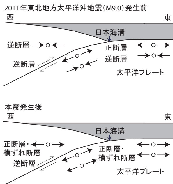
Fig. 5. 2011 年東北地方太平洋沖地震の本震発生前後の震源域内および周辺海域の応力場の変化を示した概念図. 白丸と矢印は, 上盤の陸側プレート内と太平洋プレート内の震源と地震を発生させた応力の向きをそれぞれ示す. プレート境界では, 細い矢印の向きに断層すべりが生じる逆断層型の地震が発生している.
