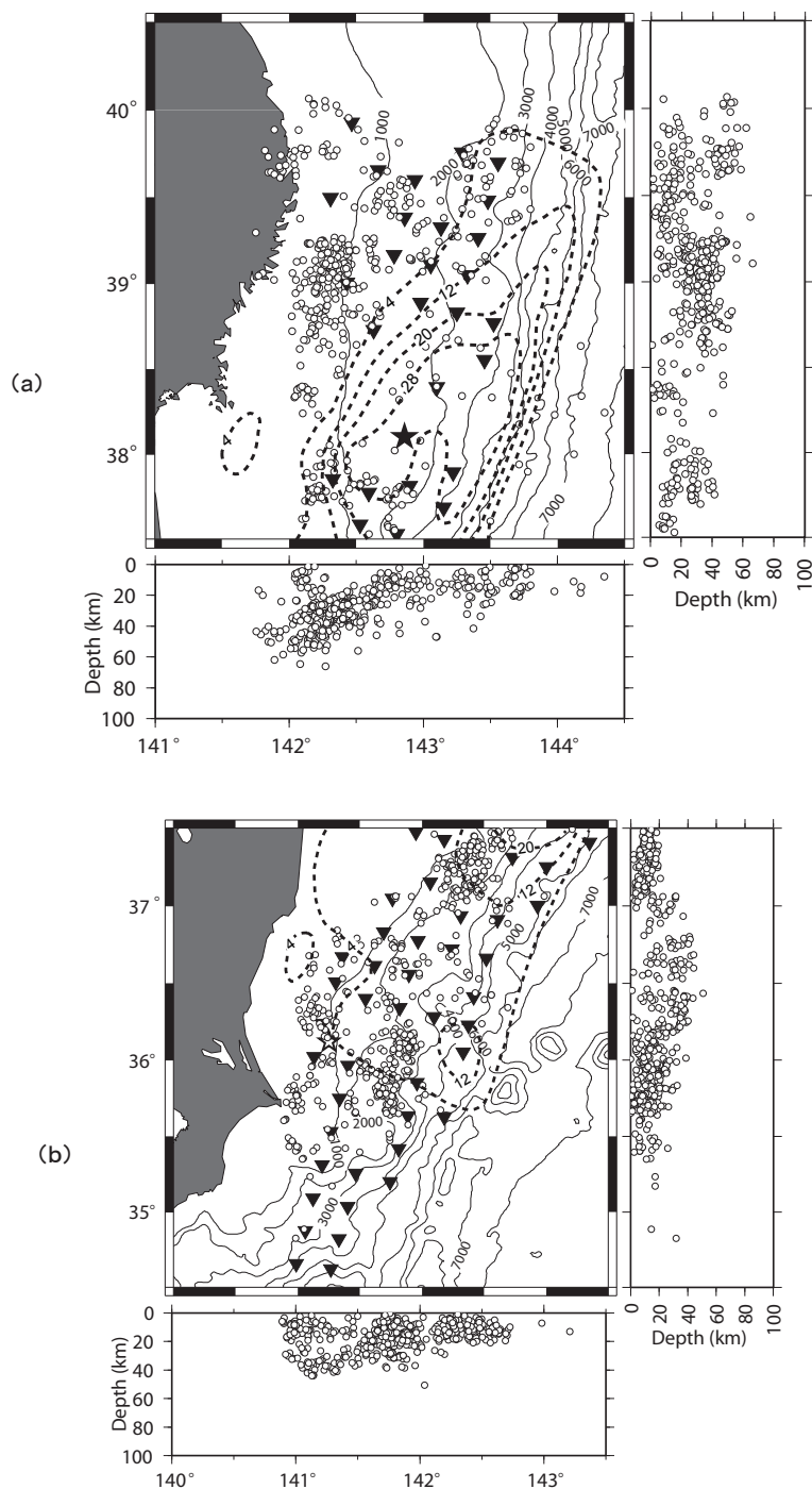
Fig. 3. 海底地震観測から求められた 2011 年 3 月 15 日から 6 月 18 日までの震源 (白丸) と, Yoshida et al. (2011) によって強震動記録から推定された本震時の断層すべり分布 (破線のコンター) との比較. 逆三角は 4 月終わりから 6 月中旬まで (第 2 期) の解析に用いた海底地震観測点を示す. 実線の等深線は水深を示す. (a) 余震域北部 (北緯 37.5 度以北) の震源分布. (b) 余震域南部 (北緯 37.5 度以南) の震源分布.
