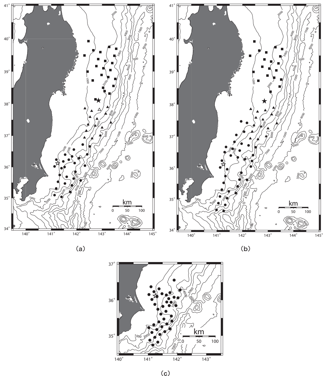
Fig. 1. 海底地震観測点分布. 四角, 三角, 丸はそれぞれ北部, 中部, 南部の解析に用いた観測点で, 白三角は中部, 南部両方の解析に用いた. 黒い星は2011年東北地方太平洋沖地震の本震(2011年3月11日14時46分, M9.0 ), 白い星は最大余震(2011年3月11日15時15分, M7.6 )の震央をそれぞれ示す. 等深線は水深を示す. (a)2011年3月14日から4月終わりまで(第1期)の観測点分布. (b)4月終わりから6月中旬まで(第2期)の観測点分布. (c)6月下旬から9月中旬まで(第3期)の余震域南部での観測点分布.
