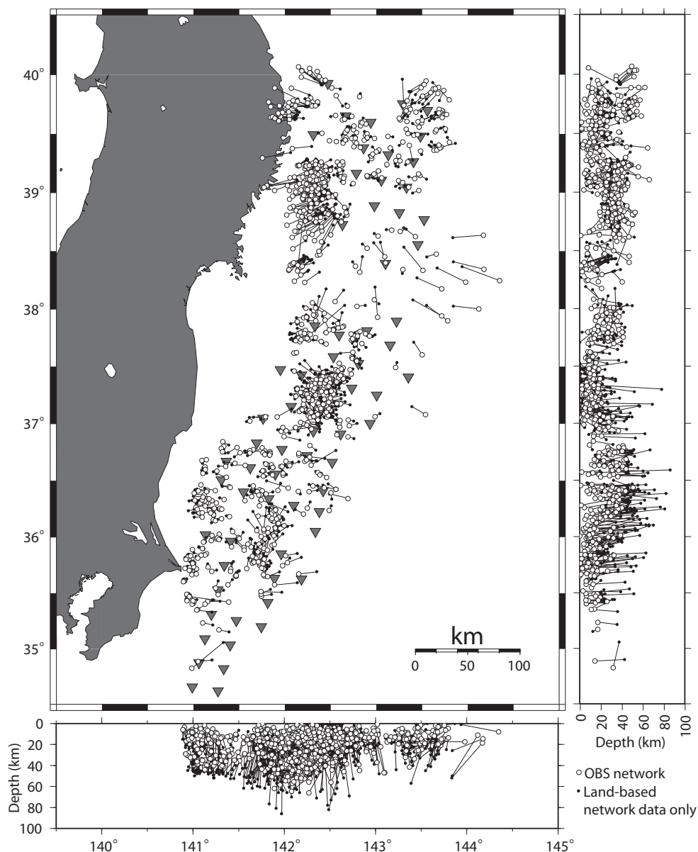
Fig. 2. 海底地震観測から求められた2011年3月15日から6月18日までの震源（白丸）と気象庁一元化震源（黒丸）との比較。逆三角は4月終わりから6月中旬まで（第2期）の解析に用いた海底地震観測点を示す。
