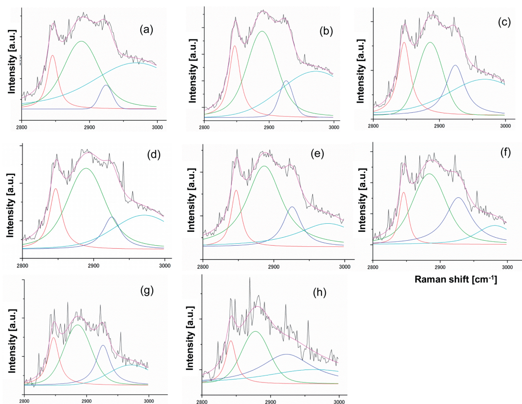
Fig. 3 : Temperature dependence of Raman spectra of DEPC liposome on the methylene C-H stretching mode: (a) 302.7\text{ K} , atmospheric pressure, (b) 303.1\text{ K} , 0.5\text{ MPa} Xe, (c) 287.5\text{ K} , 0.5\text{ MPa} Xe, (d) 285.5\text{ K} , 0.5\text{ MPa} Xe, (e) 283.2\text{ K} , 0.5\text{ MPa} Xe, (f) 281.4\text{ K} , 0.5\text{ MPa} Xe, (g) 280.2\text{ K} , 0.5\text{ MPa} Xe, (h) 278.4\text{ K} , 0.5\text{ MPa} Xe.
