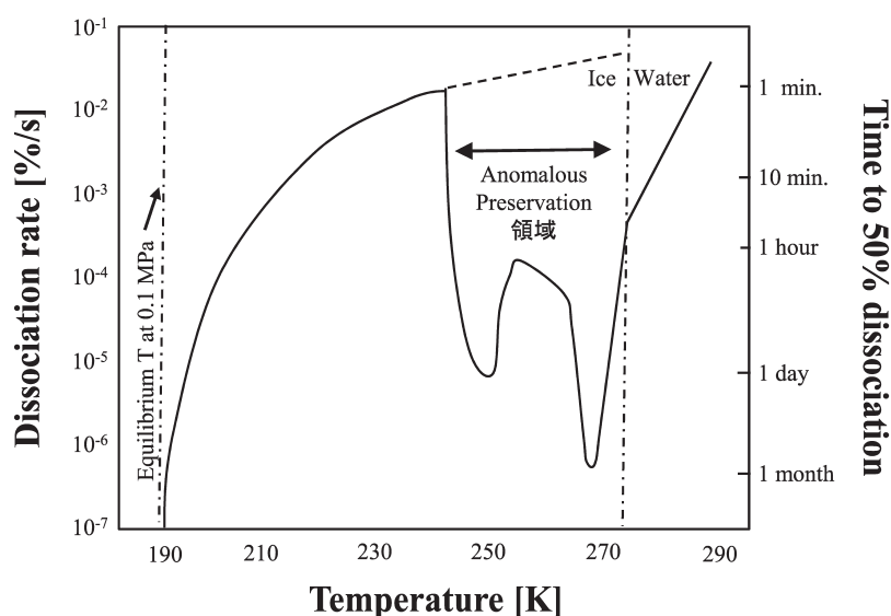
図1: Stern らにより測定された常圧メタンガス雰囲気におけるメタンハイドレートの分解速度の温度依存性 242 K–271 K の温度領域がメタンハイドレートの “Anomalous preservation” 領域 (Stern et al., 2001 をもとに作成)
