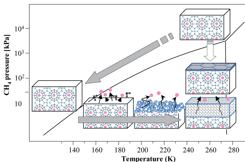
図5: ガスハイドレートの分解モデル 灰色矢印は昇温法, 白色矢印は減圧法の温度・圧力操作手順
