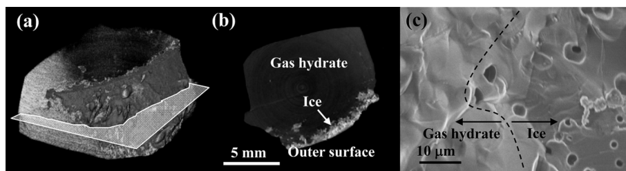
図 4：保存された天然ガスハイドレート 大気圧下の 253 K で 3 週間保存した後に測定 (a) 位相コントラスト X 線 CT 三次元像 (b) 位相コントラスト X 線 CT 二次元断面像 (c) クライオ SEM 像 (Takeya et al., 2012 をもとに作成)
