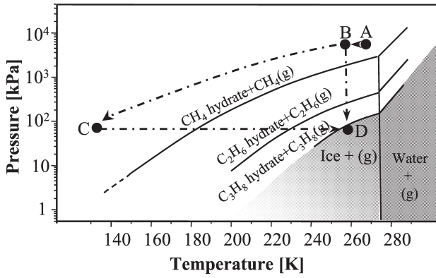
図2：メタン，エタン，プロパンハイドレートの相図 図中の灰色の部分，ガスハイドレートが安定に存在しない領域を示している
