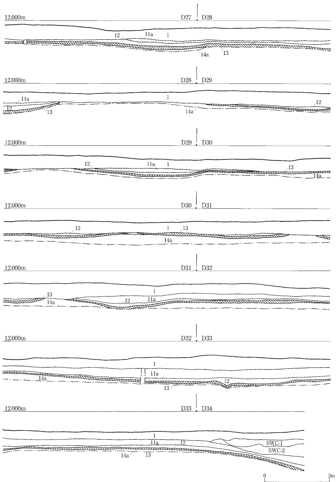
図32 西門地点トレンチⅡ北壁セクション図(5)
