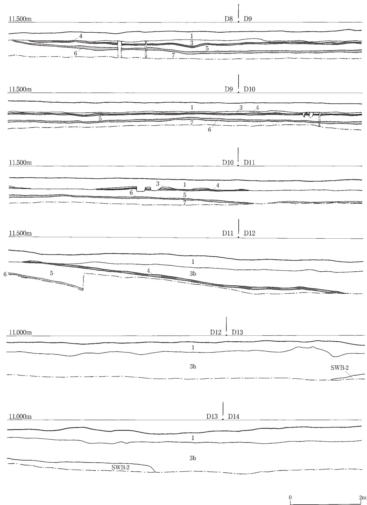
図29 西门地点トレンチII北壁セクション図(2)
