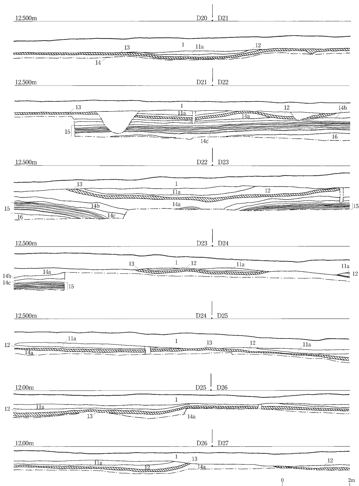
図31 西門地点トレンチⅡ北壁セクション図(4)
