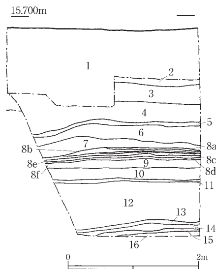
図 11 地球環境科学研究科研究棟第 2 地点 F | 西壁セクション図
