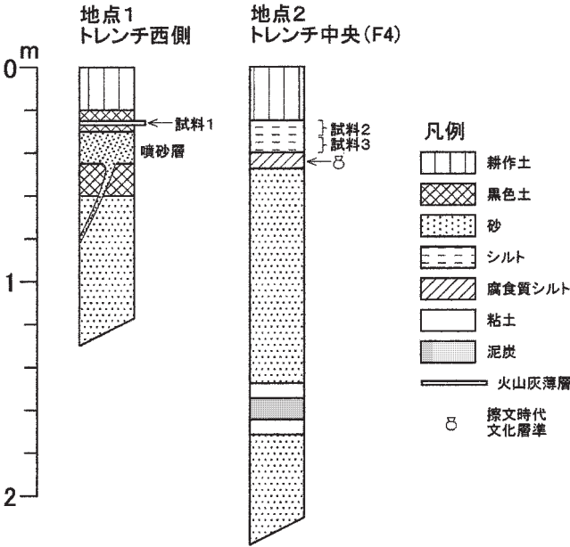
図43 西門地点試料採取地区地質柱状図
