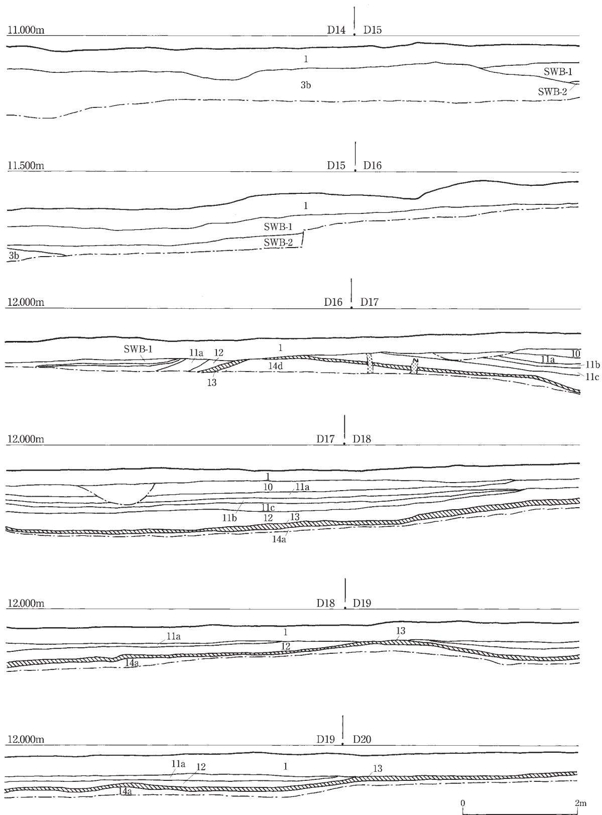
図30 西門地点トレンチⅡ北壁セクション図(3)
