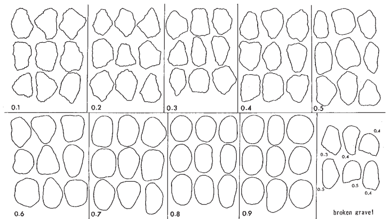
图6 円磨度印象図 (Krumbein 1941)
