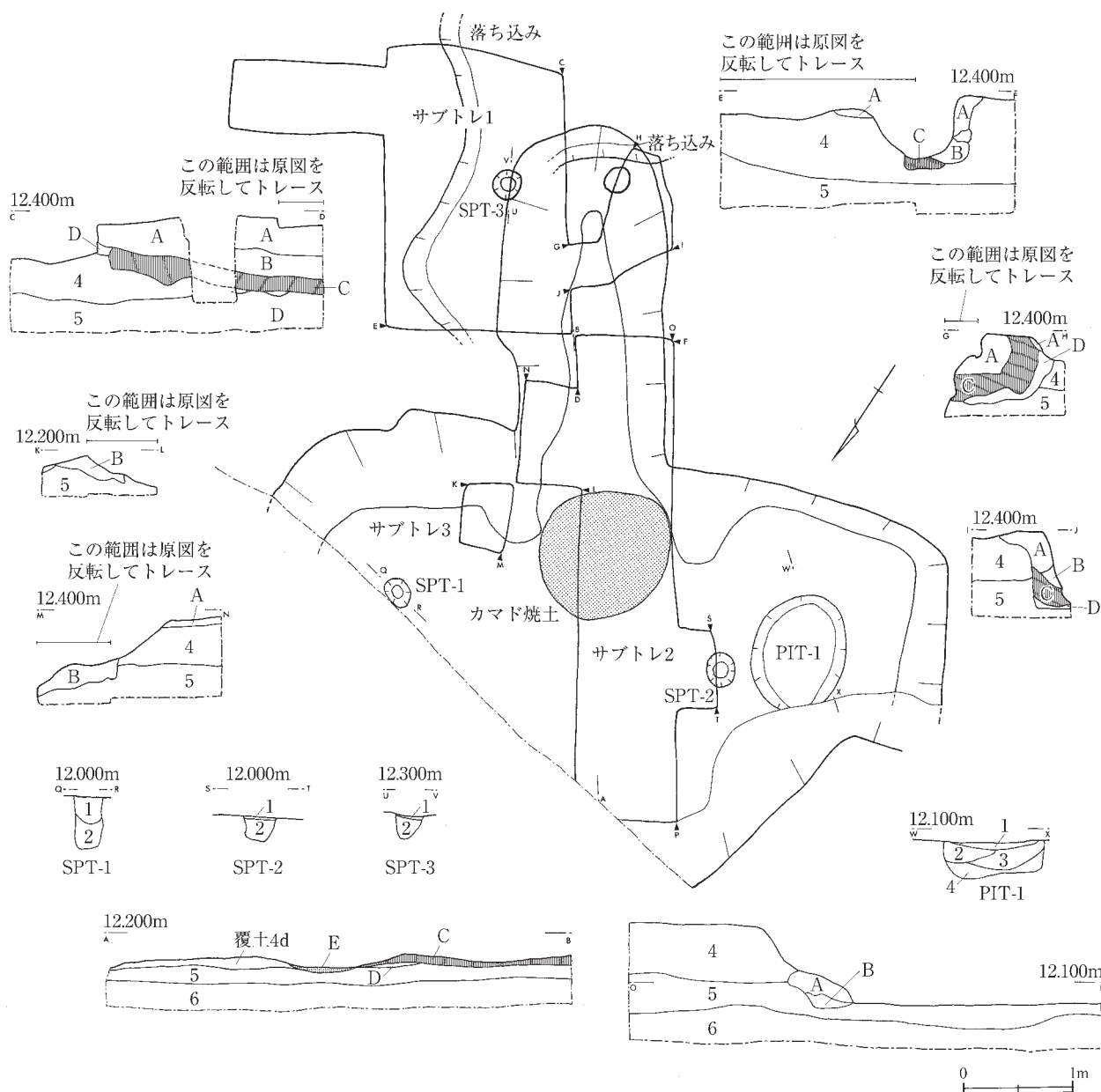
図23 工学部J・I棟間地点第I号竪穴住居址及び柱穴、土坑実測図
