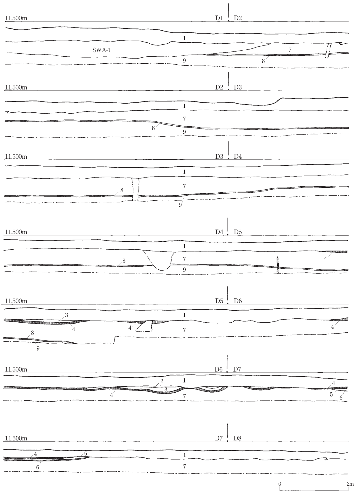
図28 西門地点トレンチⅡ北壁セクション図(I)
