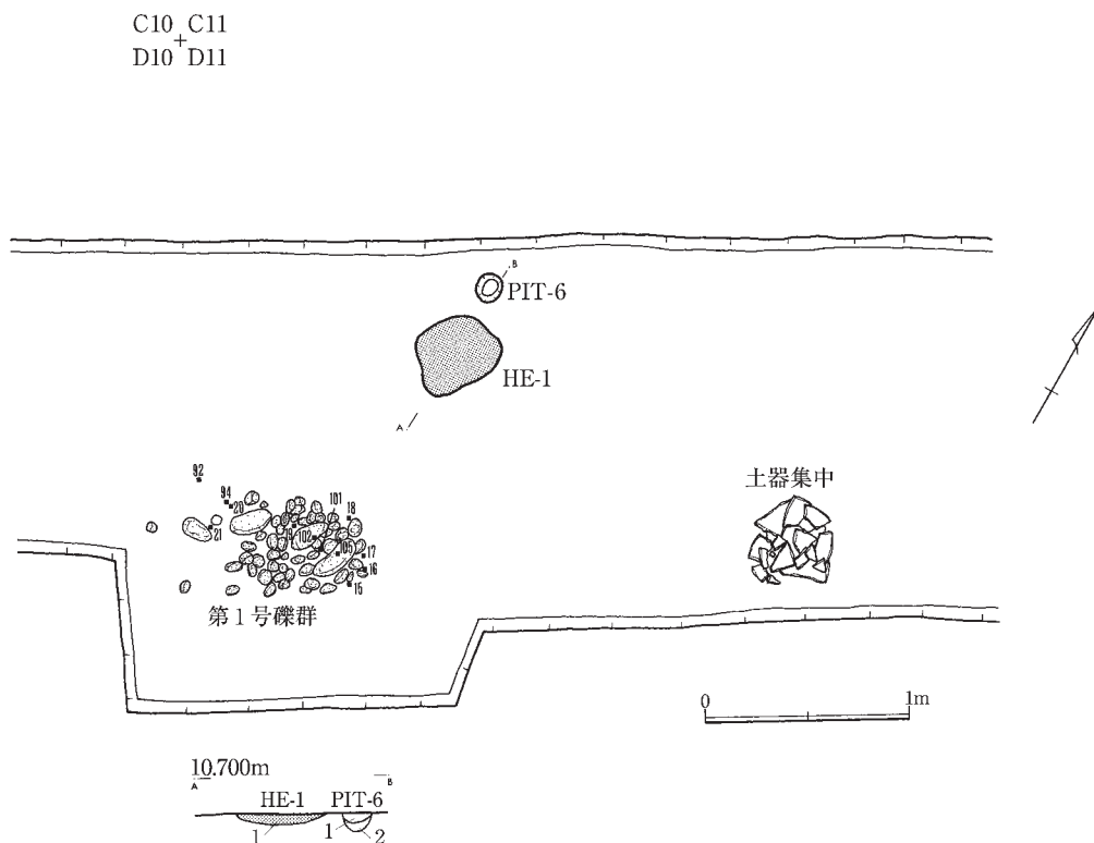
図35 西門地点 6 層出土屋外炉址（HE-I）及び第 1 号礫群実測図
