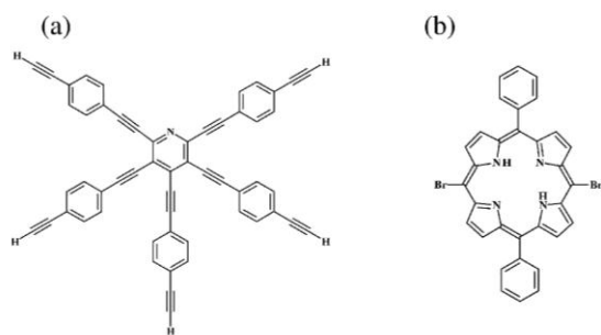
図 3. (a) pepy, (b) DBP の構造模式図。
