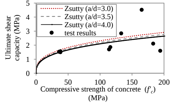
(d) Ultimate shear capacity of RC beams
