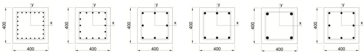
(a) ALR-24 (b) ALR-16 (c) ALR-8 (d) ALR-6 (e) ALR-4 (f) SD Serieses
