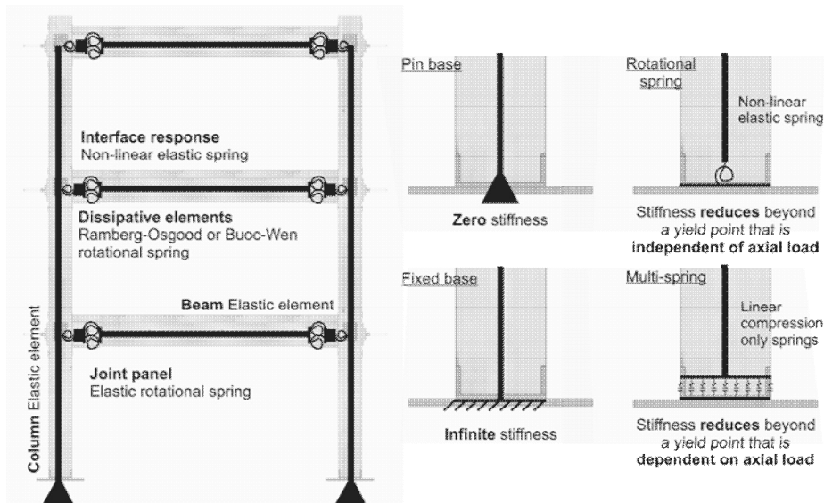
Figure 2: SAP2000 frame non linear numerical model
