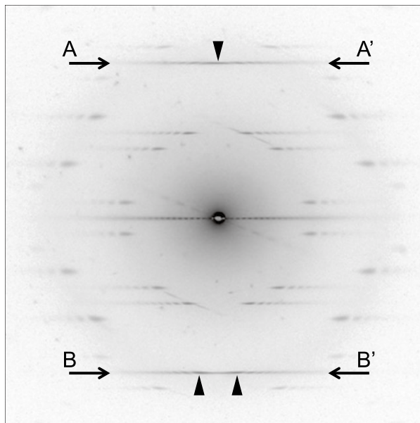
図7 単層カーボンナノチューブの回折パターン (白黒反転). (Diffraction pattern of SWCNT: reversed.)
