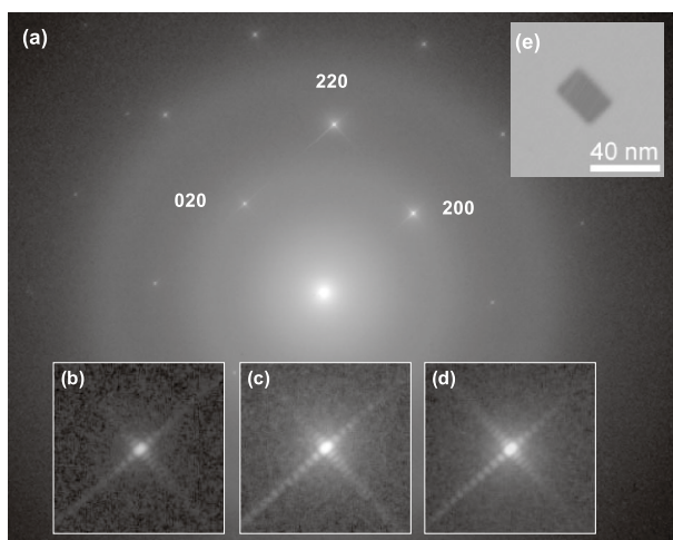
図6 MgO微粒子の回折パターンとBF-STEM像。(Diffraction pattern and BF-STEM image of MgO nanoparticle.) (a) 回折パターン全体, (b) 020 回折スポット, (c) 220 回折スポット, (d) 200 回折スポット, (e) BF-STEM 像.
