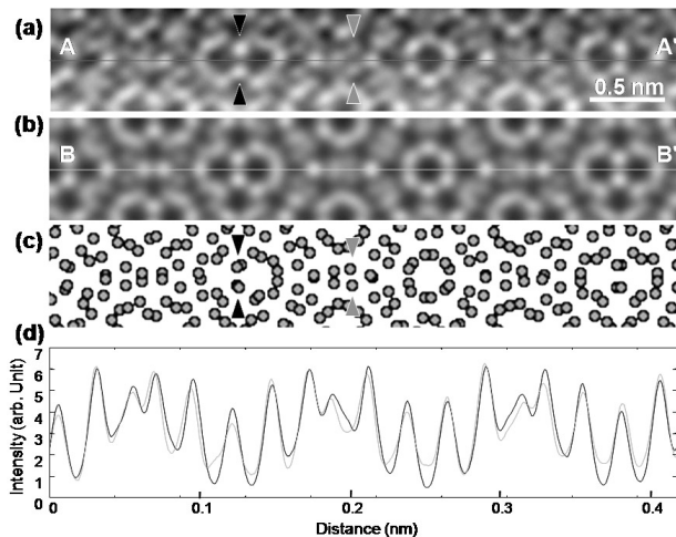
図9 単層カーボンナノチューブでの原子分解能化回折イメージング実証結果. (Verification of atomic-resolution diffractive imaging.) (a) 再構成像, (b) シミュレーション結果, (c) 原子配列モデル, (d) ラインプロファイル比較.
