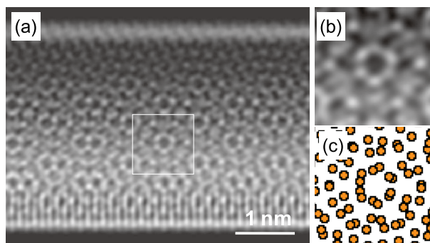
図8 単層カーボンナノチューブ再構成像。(Reconstructed pattern of SWCNT.)
