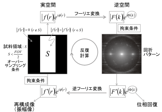
図2 フーリエ反復位相回復法概念図。(Schematic diagram of iterative phase retrieval.)
