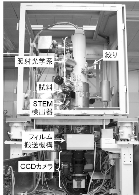
図4 電子回折顕微鏡概観図。（Appearance of electron diffraction microscope.）
