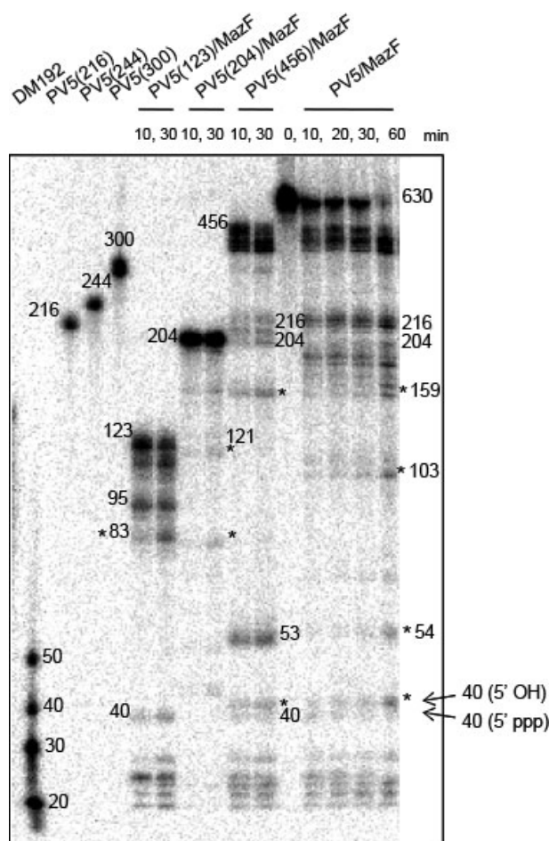
Fig.3.2.3 PV5 の MazF による切断産物
