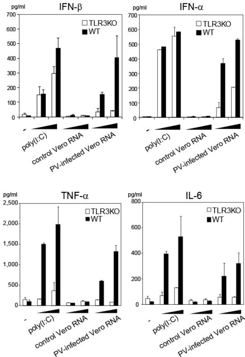
Fig.1.1 ポリオウイルス感染細胞由来の RNA による TLR3 依存的なサイトカイン産生
