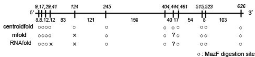
Fig.3.2.2 PV5 の二次構造モデルによる MazF 切断サイトの感受性の比較
