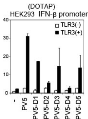
Fig.3.4.2 PV5 欠損体エンドソーム直接送達による IFN-βプロモータの活性化
