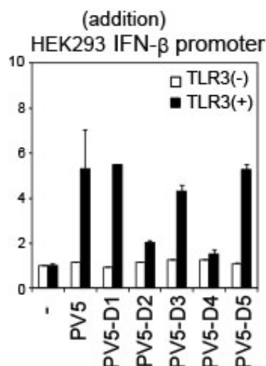
Fig.3.4.1 PV5 欠損体による IFN-βプロモータの活性化
