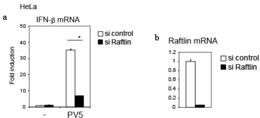
Fig.2.6.2 PV-RNA による TLR3 依存的 IFN-βプロモータの活性化における Raftlin の関与
