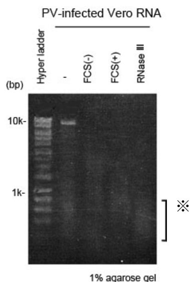
Fig.1.3.1 ポリオウイルス感染細胞由来の RNA の血清中での安定性
