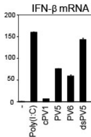
Fig.2.3.2 PV-RNA による IFN- \beta mRNA 誘導
