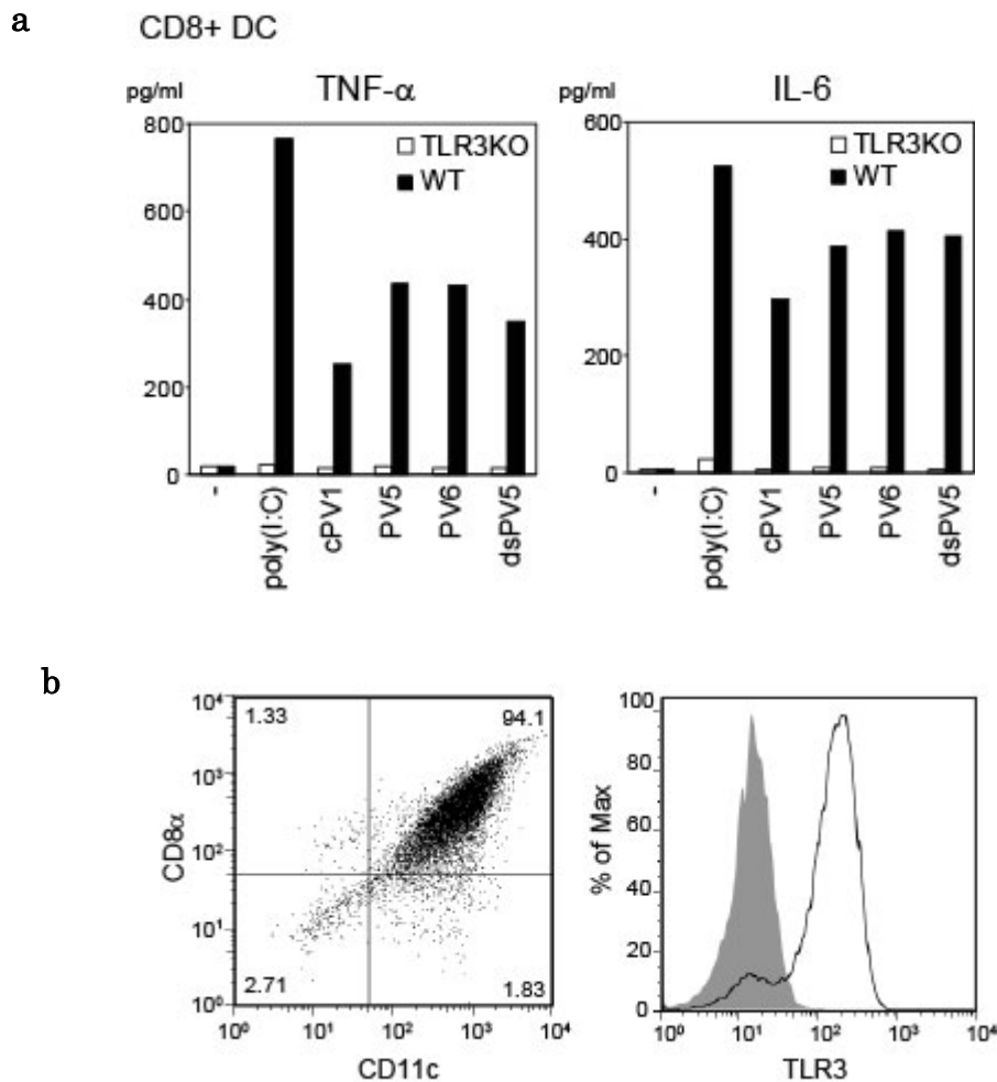
Fig.2.8.3 マウス CD8 陽性樹状細胞における、PV-RNA によるサイトカイン産生
