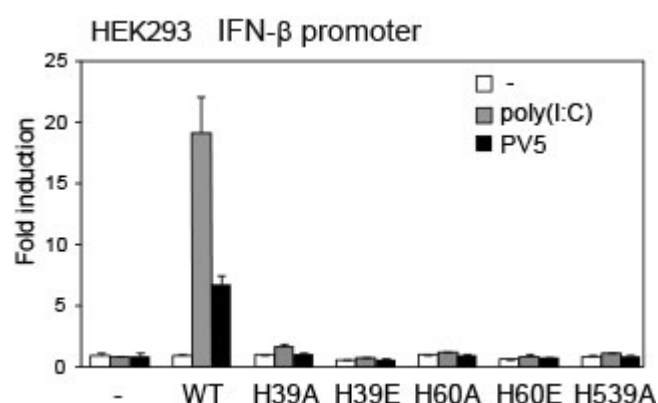
Fig.2.5 PV5 刺激における TLR3 のリガンド結合変異体発現の影響
