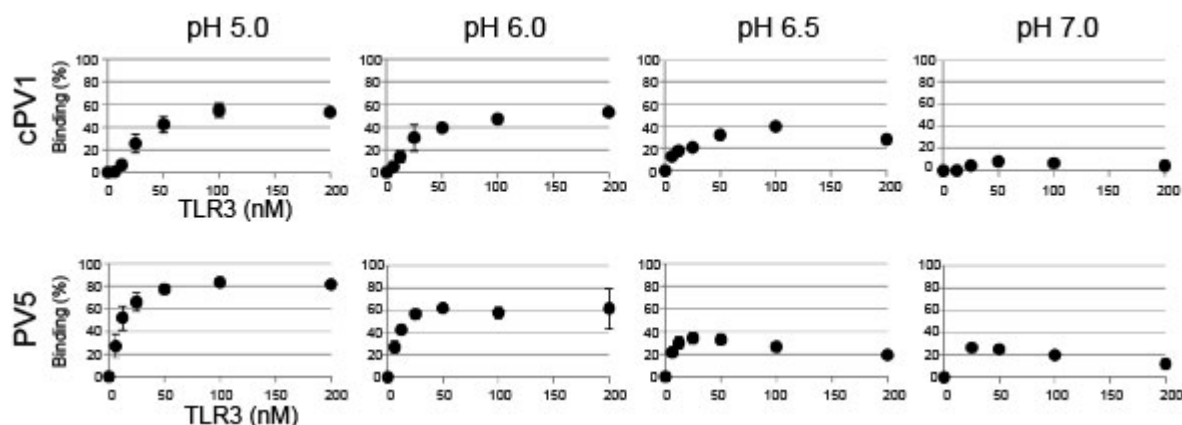
Fig.2.4 PV-RNA と TLR3 の結合性
