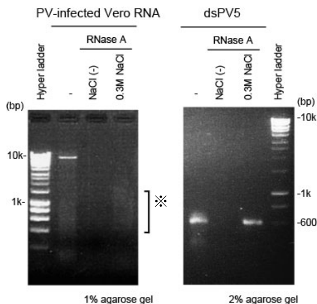
Fig.1.3.2 ポリオウイルス感細胞由来の RNA に含まれる ssRNA
