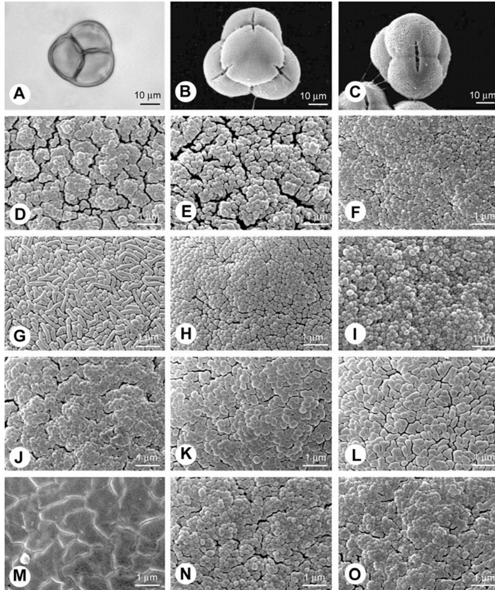
Fig. 1. LM and SEM micrographs of Rhododendron pollen. A) R. formosanum (Murata 17561); B) R. maddenii (Kanai et al. 346?); C) R. tsusiophyllum (Sawada s.n.); D) R. aureum (Takahashi 2512); E) R. kaempferi (Iketsu et al. 95); F) R. aureum (Takahashi 2512); G) R. brachycarpum (Takahashi et al. 40); H) R. decorum (Smith 2016); I) R. degonianum (Iketsu 1763); J) R. formosanum (Murata 17561); K) R. macrostemon (Togasi 688); L) R. viscistylum var. amakusaense (Minamidani 29613); M) R. semibarbatum (Murata 7987); N) R. arborescens (Unknown s.n.); O) R. albrechtii (Takahashi 3975). Pollen tetrads at polar view (A-D); tetrads with viscin threads (A, B, D); pollen tetrad at equatorial view with viscin threads (E); micrographs with apocolpial exine sculpture details (F-O).
