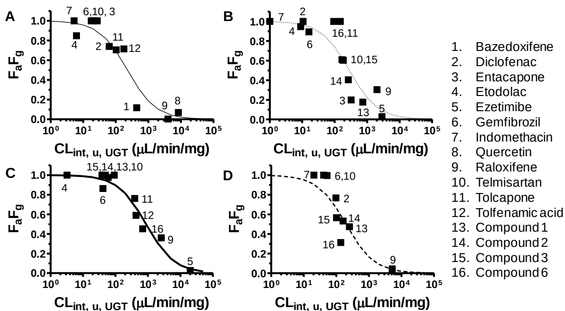
図 3-3. 評価化合物のヒト (A), ラット (B), イヌ (C), およびサル (D) における F_aF_g と CL_{int,UGT} の関係
