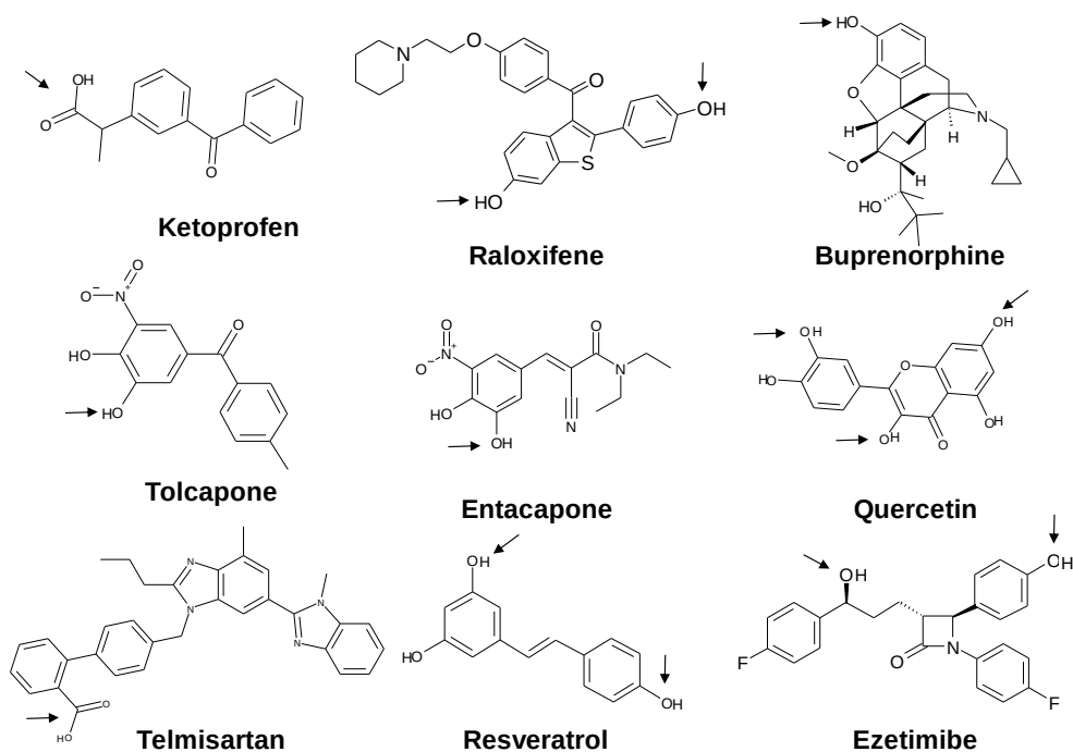
図 2-1. 評価化合物の構造
