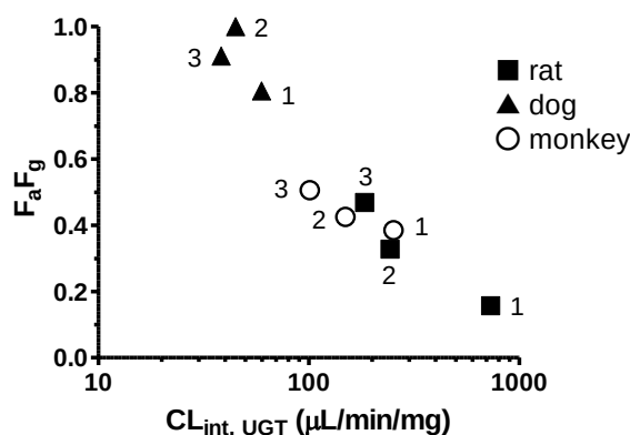
図 1-4. 化合物 1-3 の F_aF_g と CL_{int,UGT} の関係
