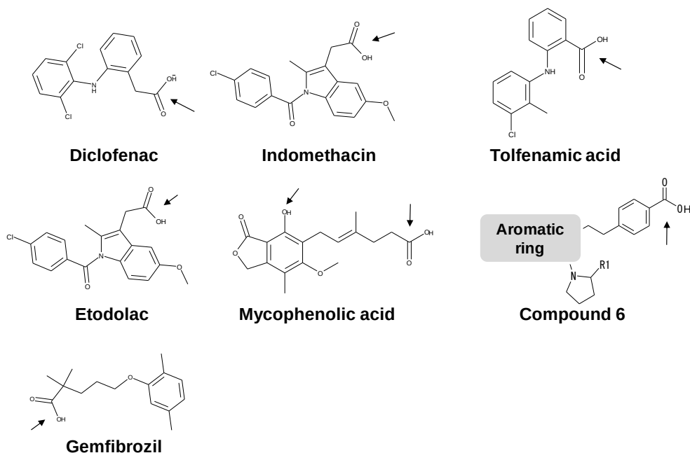
図 3-1. 評価化合物の構造
