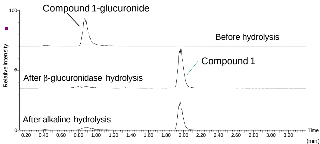
図 1-3. 化合物 1 投与後のラット胆汁中の LC-MS/MS クロマトグラム
