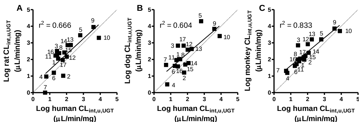
図 3-2. ヒト, ラット, イヌ, およびサルの CL_{int,u,UGT} の比較
