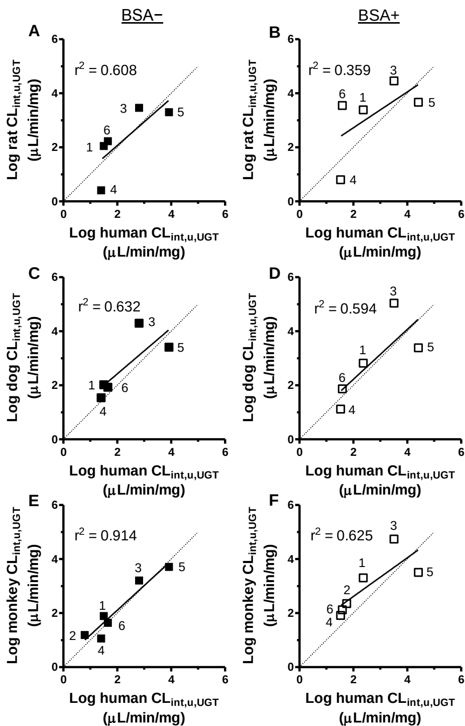
図 3-6. 小腸マイクロソーム中の CL_{int,u,UGT} のヒトとラット, イヌ, およびサルと比較
