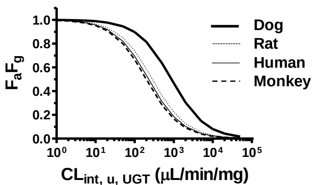
図 3-4. CL_{int,u,UGT} と F_aF_g の関係の動物種間比較
