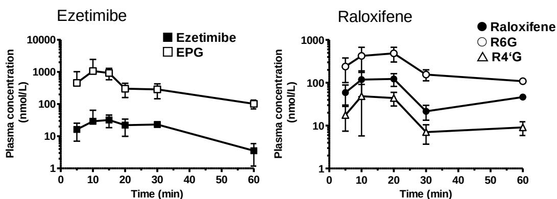
図 2-2. 経口投与後の門脈血漿中の未変化体およびグルクロン酸抱合体の濃度推移 (平均値±標準偏差, n = 3-4)
