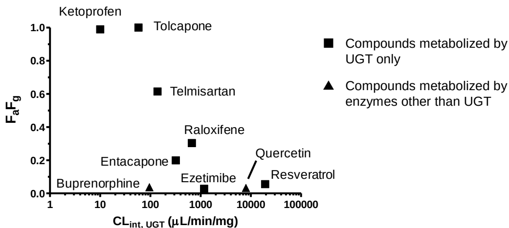
図 2-3. ラットにおける UGT 基質の CL_{int,UGT} と F_a F_g の関係
