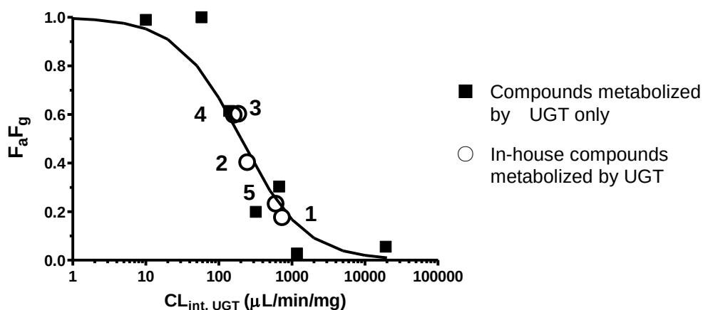
図 2-4. SIA モデルによるフィッティングカーブと化合物 1-5 の CL_{int,UGT} と F_a F_g の関係
