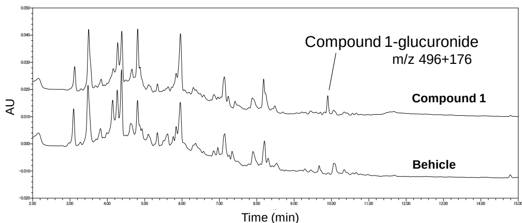
図 1-2. 化合物 1 または投与溶媒のみを投与後 0-6 時間のラット胆汁の LC-UV クロマトグラム
