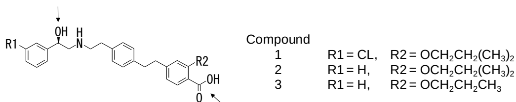
図 1-1. 新規カルボン酸化合物 1-3 の構造
