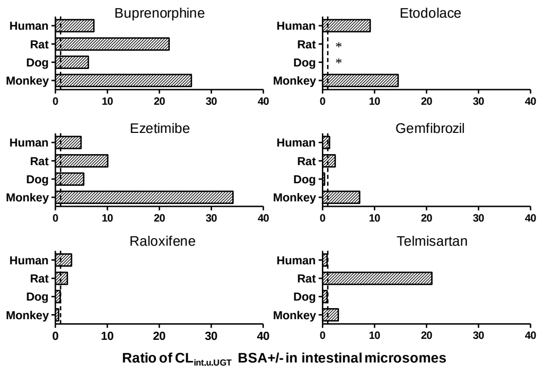
図 3-5. BSA 添加条件／非添加条件におけるヒト、ラット、イヌ、およびサル小腸マイクロソーム中の CL_{int,u,UGT} の比
