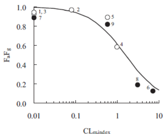
図 序-1. CYP3A 基質の F_a F_g と CL_{m, index} (評価化合物とリファレンス化合物の CL_{int,CYP} の比) の関係 曲線は SIA モデルによるフィッティングカーブを示す。
