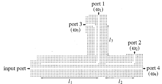
Fig. 13. Four-channel MUX-DEMUX.
