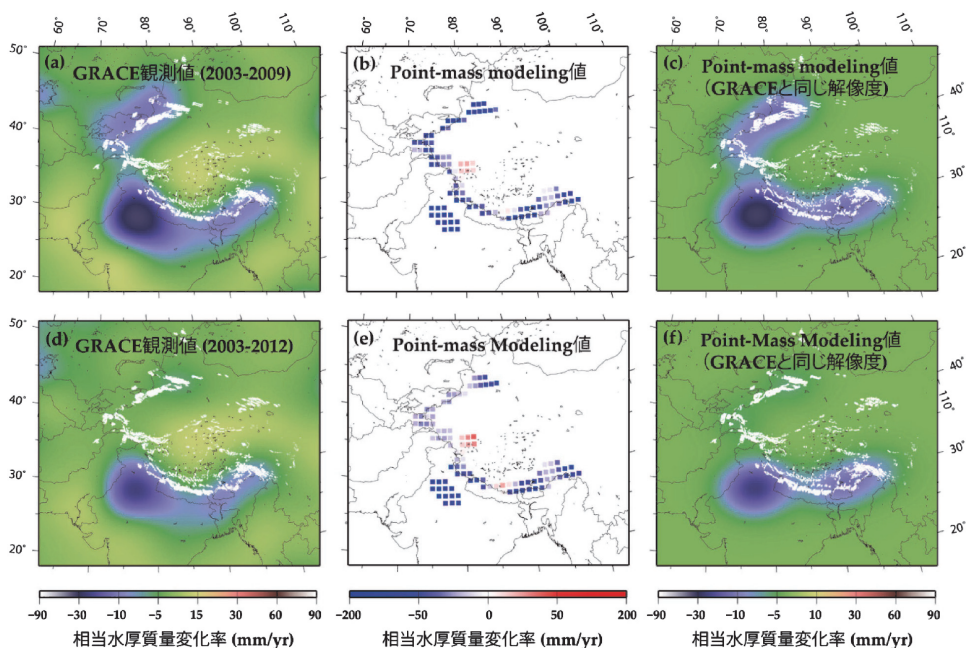
図 2 (a) GRACE で観測された 2003-2009 年の質量経年変化. なお, 氷河周辺の陸水変動 (深さ \sim 5 m まで) は, 陸水モデル GLDAS によって補正済みである. (b) (a) の GRACE の観測データを基に, Point-mass modeling 法によって導かれた 2003-2009 年の氷河質量変化率および地下水変化率. (c) (b) の結果に GRACE と同じ空間フィルター (半径 300 km の非等方ガウシアンフィルター) を施したもの. (c)-(f) (a)-(c) を 2003-2012 年で行ったもの.
