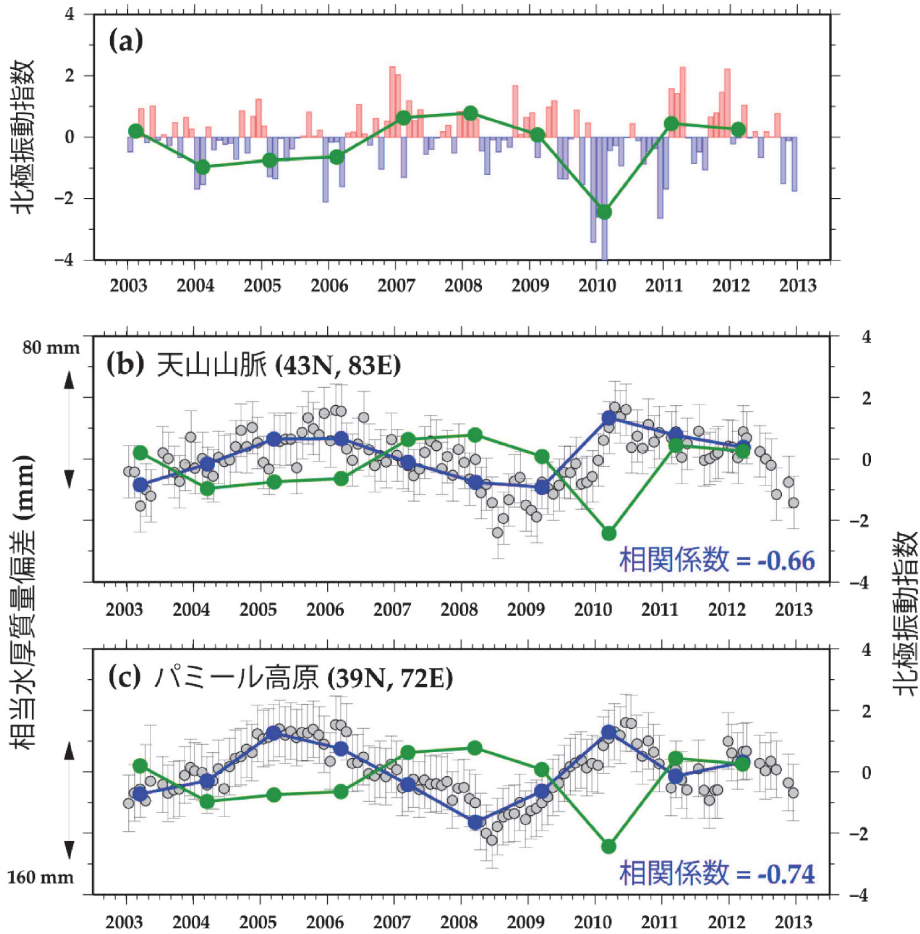
図 3 (a) 月毎の北極振動指数の時系列。データは、アメリカ海洋大気庁により入手した。( http://www.cpc.ncep.noaa.gov/products/precip/CWlink/daily_ao_index/ao.shtml )。赤と青のバーは、それぞれ正の北極振動、負の北極振動を示す。緑の曲線は、冬期 (1-3 月) の平均をとったもの。 (b) 天山 (43N, 83E) における相当水厚質量偏差 (EWD) の時系列。青の曲線が、冬期の 3ヶ月平均を示す。右下に冬期の EWD (青の曲線) と北極振動 (緑の曲線) の相関係数を示す。 (c) パミール (39N, 72E) における EWD 時系列。
