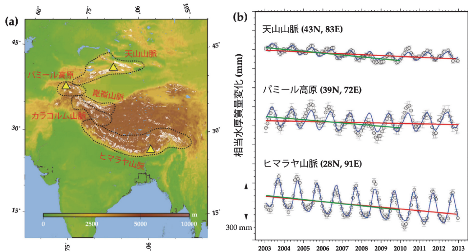
図 1 (a) アジア高山域の山岳氷河群の地理的分布. 白色のドットが氷河領域を示す. ここでは, ヒマラヤ山脈 (28N, 91E), カラコルム山脈 (36N, 75E), 崑崙山脈 (36N, 80E), パミール高原 (39N, 72E), 天山山脈 (43N, 83E) が有する氷河群について解析する. それぞれの氷河群を黒の破線で囲む. (b) GRACE RL05 データから導かれた, 天山, パミール, ヒマラヤの相当水量質量 (EWT) 変化の時系列 (図 1a の黄色い三角で示した点). エラーバー ( 1\sigma ) のついた白丸が, GRACE から観測された EWT 変化を表す. 赤の直線は, 最小二乗法によって得られた 2003-2012 年の質量経年 (1 次) 変化, 緑の直線が, 2003-2009 年の 1 次変化, 青の曲線が, 平均的な季節 (年周+半年周) 変化を示す.
