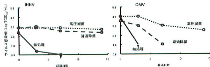
図 2. 魚類飼育水中における IHNV および OMV の生存性 (15℃)。
