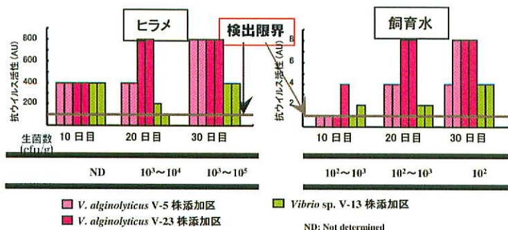
図6. 抗ヘルペスウイルス活性を有する V. alginolyticus V-5 株, V-23 株投与時のヒラメ腸内容物および飼育水の抗ウイルス活性。
