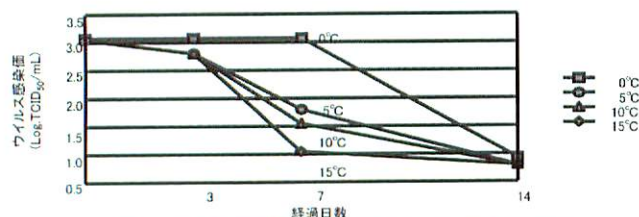
図 1. 魚類飼育水中での IHNV ウイルスの生存性。
