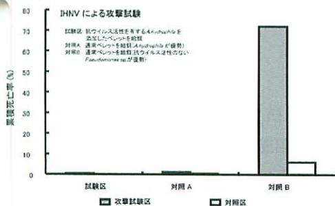
図3. 抗 IHNV 活性を有する腸内細菌 Aeromonas hydrophila M-36 株を添加したペレットを給餌したサクラマスの死亡率。
