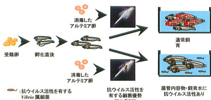
図4. 抗ウイルス活性を有する細菌を用いたマツカワのウイルス性神経壊死症制御の試み。
