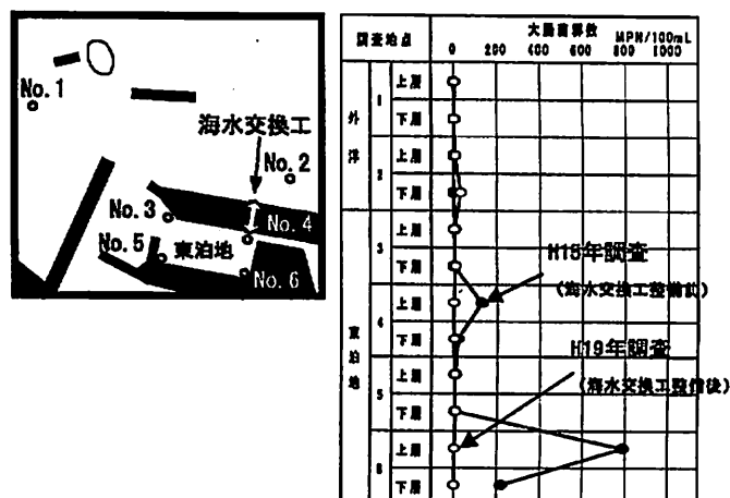
図-7 防波堤改良による水質の変化
