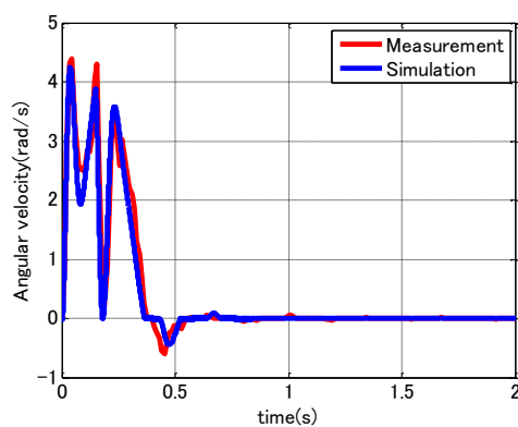
(a) モータの角速度
