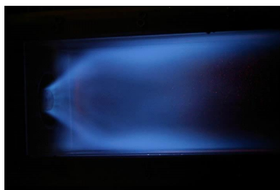
(e) 2次火炎ありのときの火炎の様子
