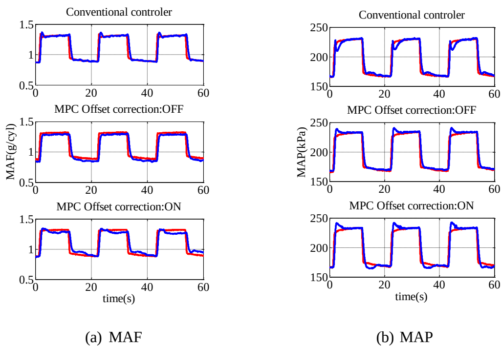
図 4.27 ステップ応答(2400rpm, 40 mm 3 /st → 80 mm 3 /st)
