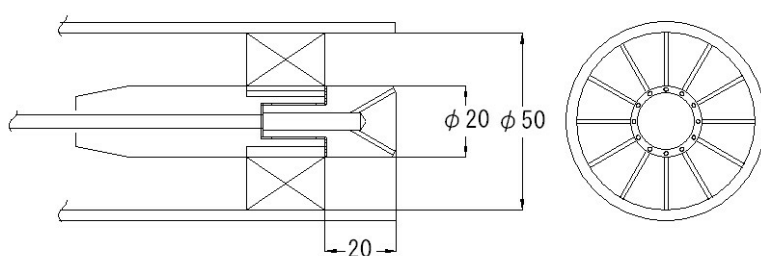
(b) スワラの形状
