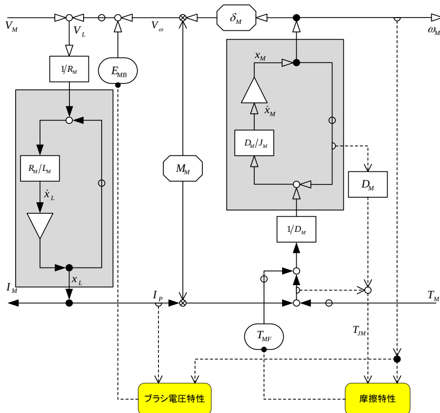
図 3.18 モータのモデル(変形)
