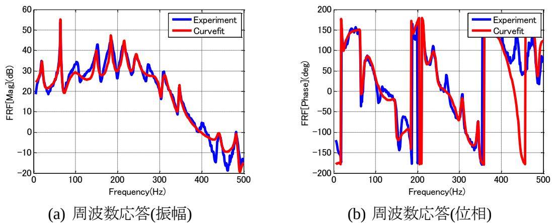
図 2.5 実験結果およびカーブフィット結果(当量比:0.25, シミュレーション用)
