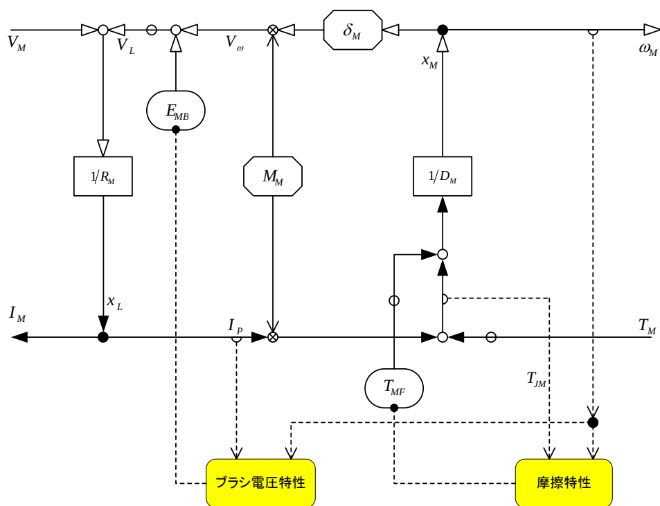
図 3.19 モータの定常モデル
