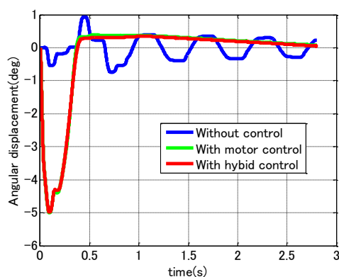
(c) モータ 2 の角変位
