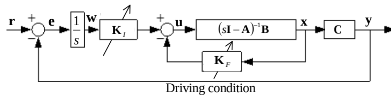
図 4.9 適応制御系
