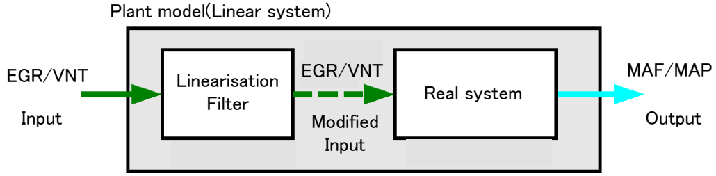
図 4.4 線形化フィルタを含むプラントモデル
