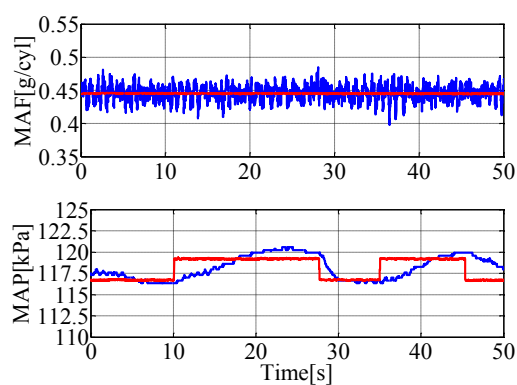
(b) MAP 目標値を変化させた 場合の応答
