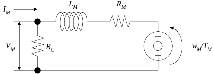
図 3.15 モータの回路
