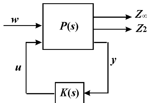
図 2.2 混合 H_2/H_\infty 最適化問題
