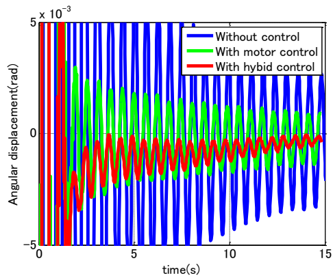
(e) 梁 1 先端の角変位(拡大)
