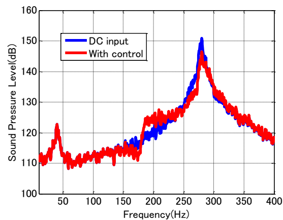
図 2.19 シミュレーション結果
