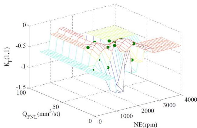
図 4.10 フィードバックゲインマップ
