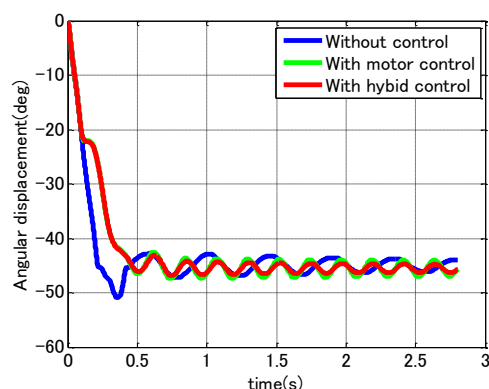
(a) モータ 1 の角変位
