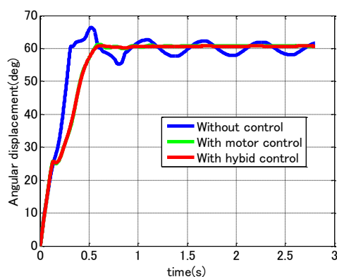
(a) モータ 1 の角変位
