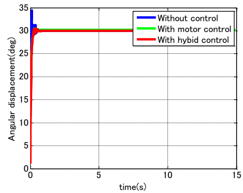
(b) モータ 2 の角変位
