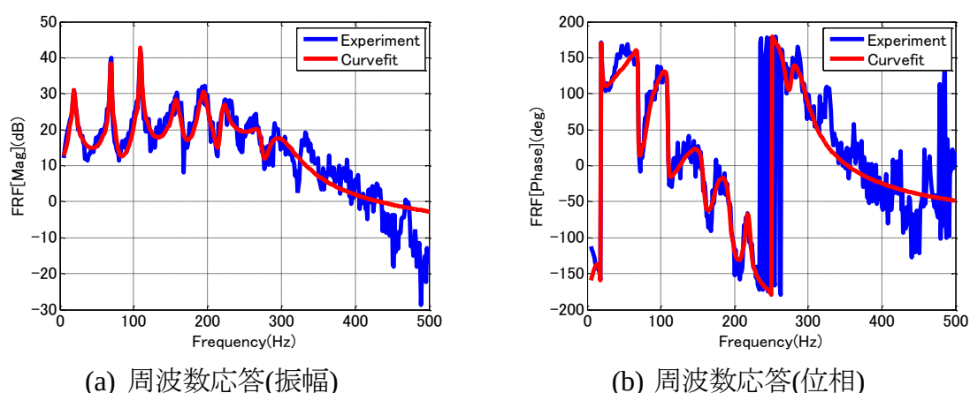
図 2.10 実験結果およびカーブフィット結果(当量比 : 0.39, 設計用)
