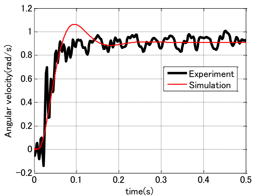
図 3.20 ステップ応答(3.0V)
