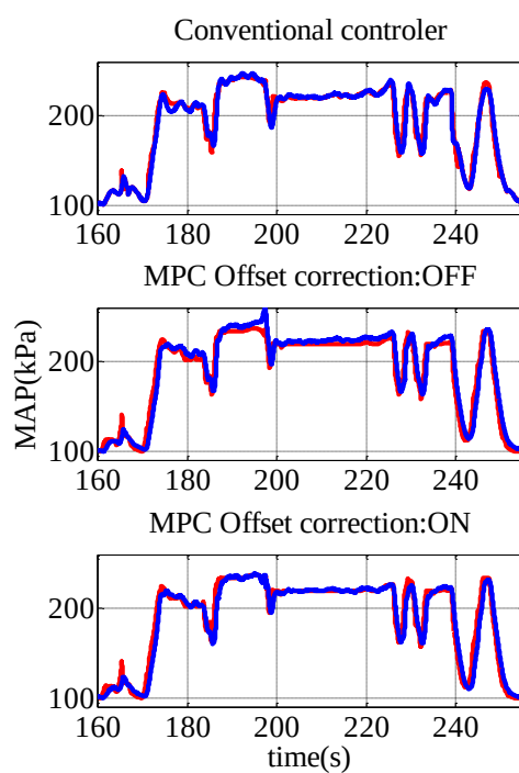
(d) MAP
