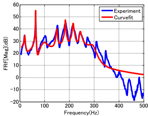
(a) 周波数応答(振幅)
