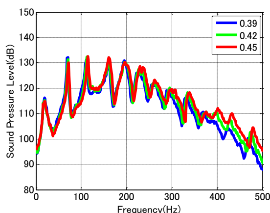
図 2.15 制御下での高い当量比における音圧レベル
