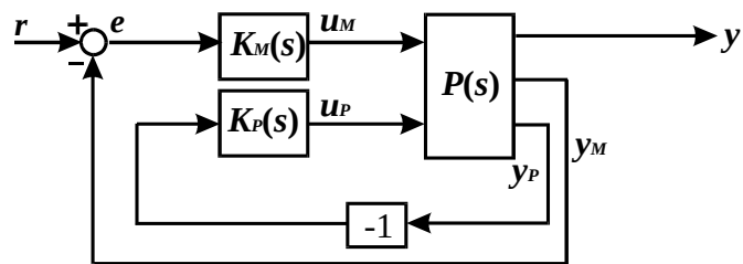
図 3.39 運動および振動に関する制御系のブロック線図
