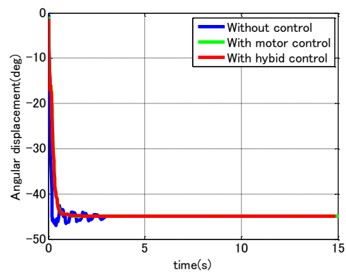
(a) モータ 1 の角変位
