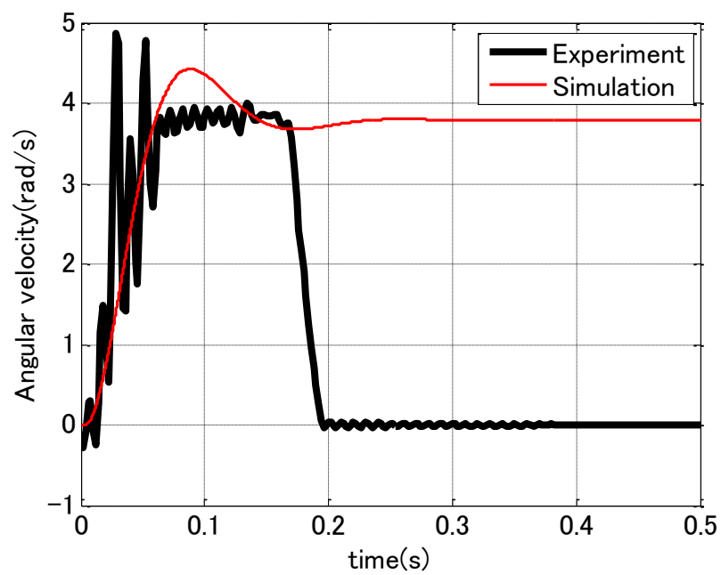
図 3.22 ステップ応答(7.0V)
