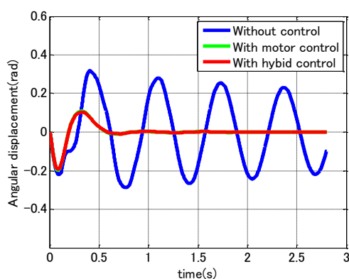
(c) 梁 1 先端の角変位
