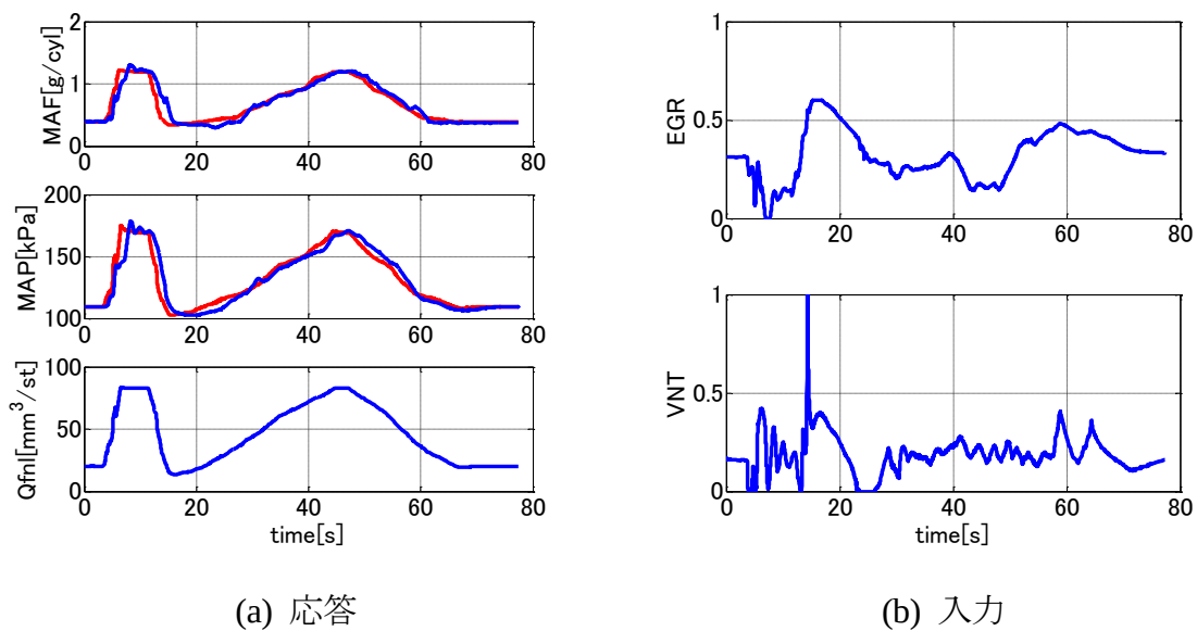
図 4.17 マッピングによる適応制御性能実験結果(1500rpm, 20-80mm 3 /st)
