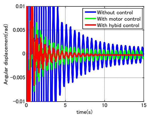
(e) 梁 1 先端の角変位(拡大)
