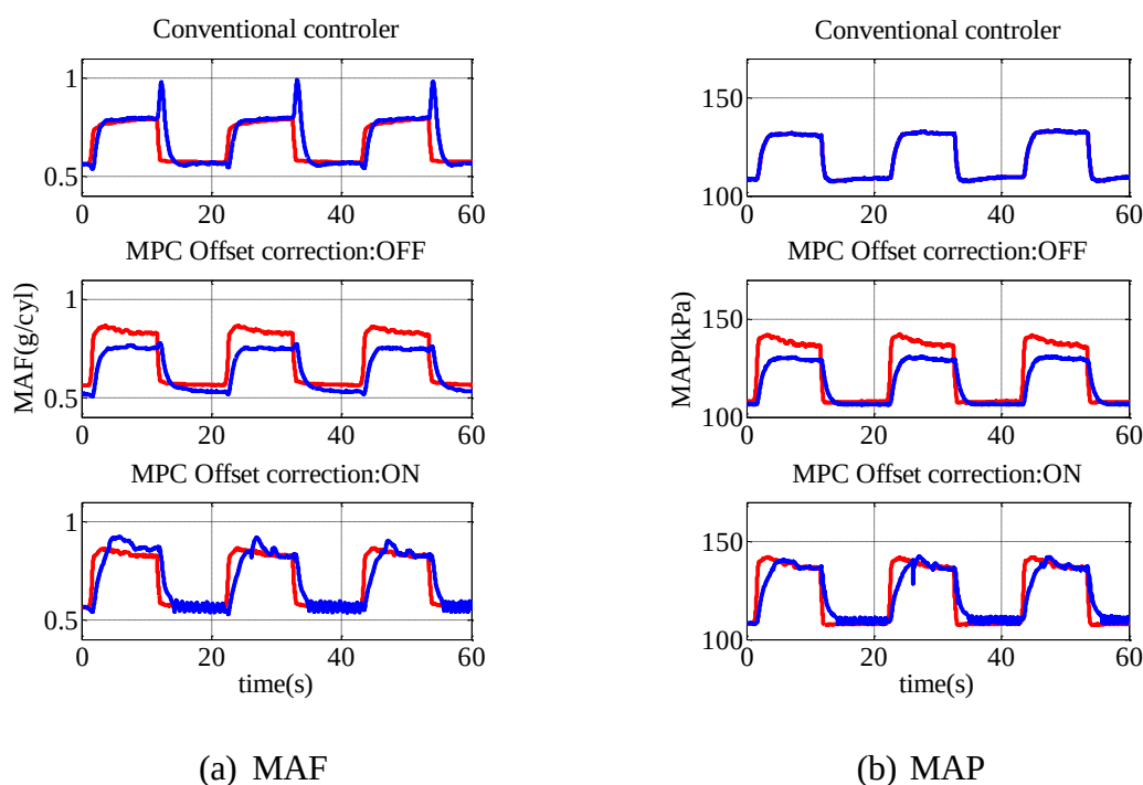
図 4.21 ステップ応答(1200rpm, 10 \text{ mm}^3/\text{st} \rightarrow 40 \text{ mm}^3/\text{st} )
