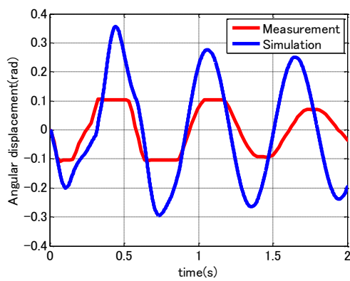
(c) 梁 1 先端の角変位
