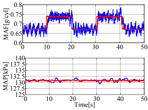
(c) MAF 目標値を変化させた 場合の応答 (実験結果)
