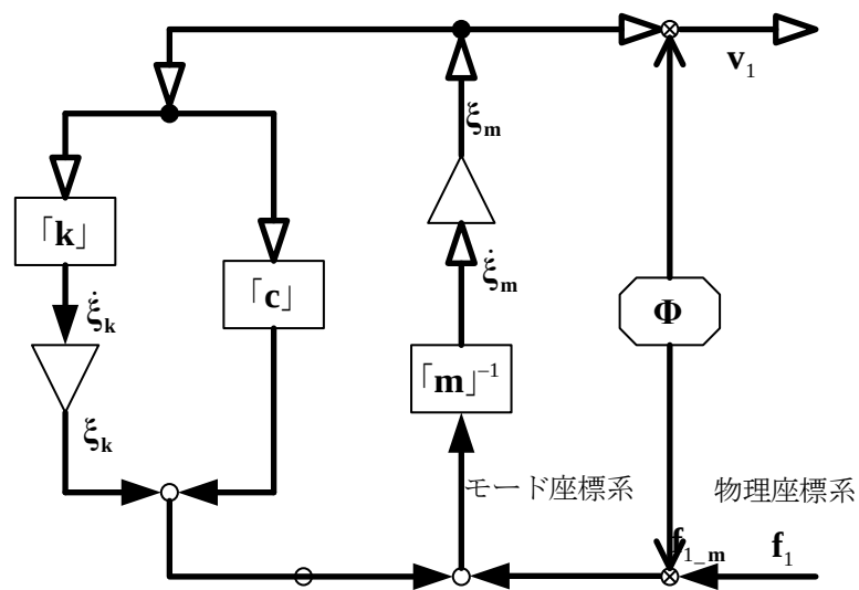
図 3.26 モード座標に変換する機能モデル
