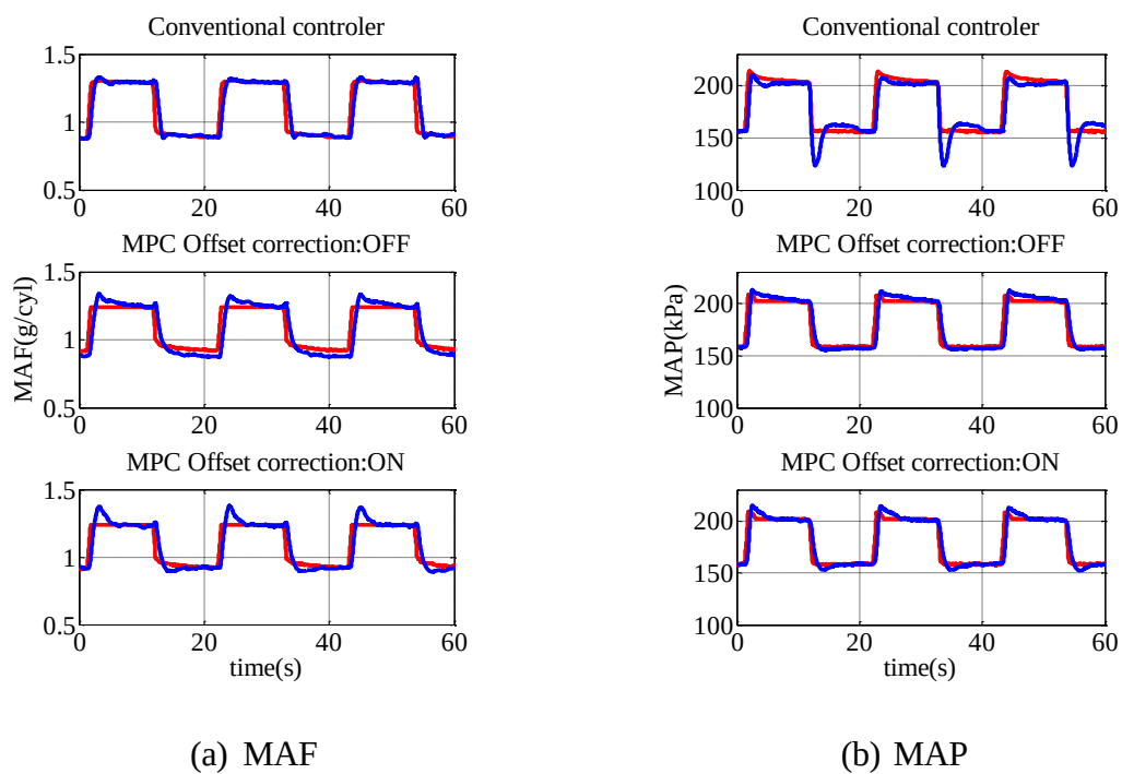
図 4.23 ステップ応答(1600rpm, 40 \text{ mm}^3/\text{st} \rightarrow 80 \text{ mm}^3/\text{st} )
