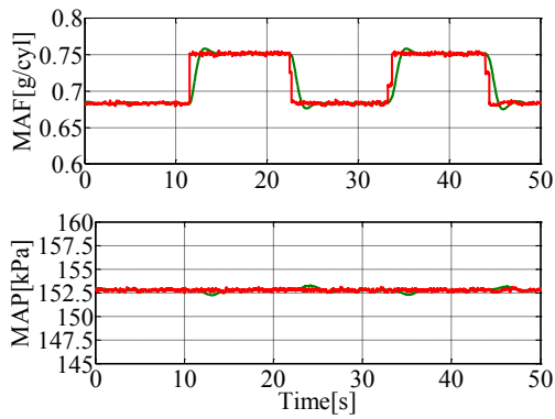
(a) MAF 目標値を変化させた 場合の応答 (シミュレーション結果)
