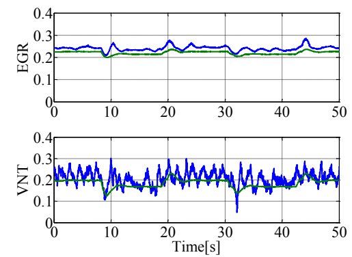
(f) MAP 目標値を変化させた 場合の入力
