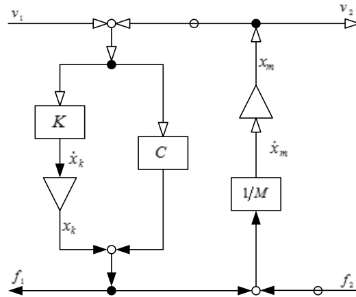
図 3.24 1 自由度系の機能モデル
