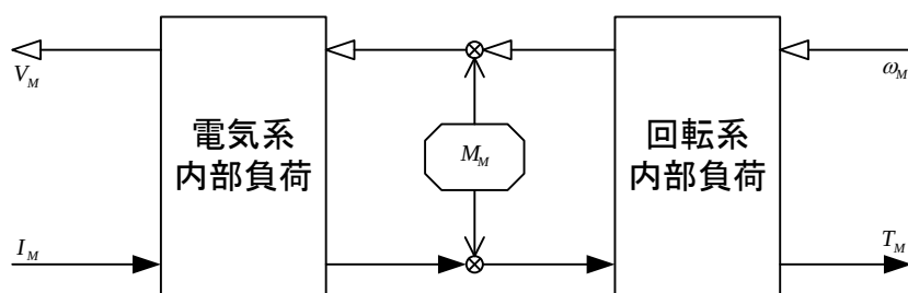
図 3.14 モータ機能モデル(基本型)
