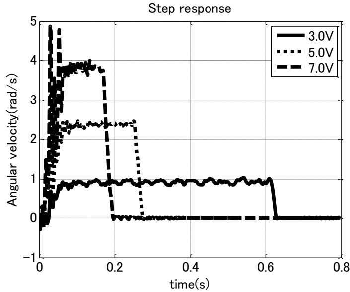
図 3.17 モータのステップ応答
