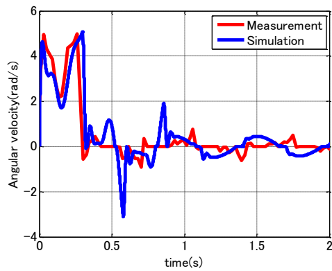
(a) モータ 1 の角速度
