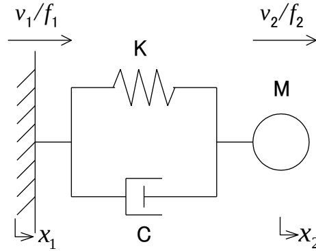
図 3.23 1 自由度系の構造モデル
