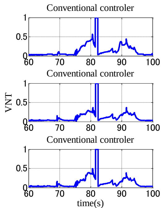
(b) VNT 指示開度
