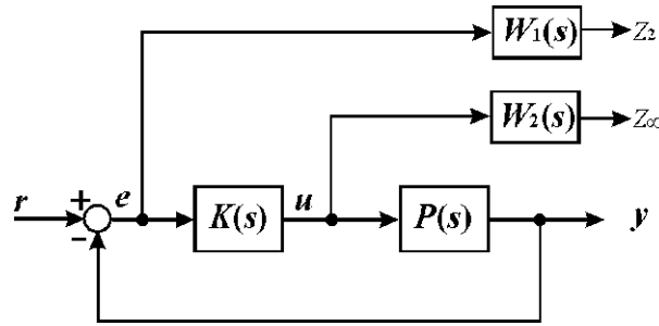
図 3.38 制御系のブロック線図
