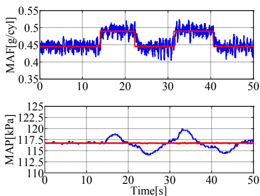
(a) MAF 目標値を変化させた 場合の応答
