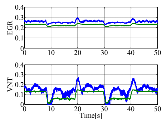
(f) MAF 目標値を変化させた 場合の入力
