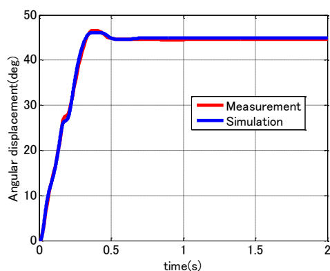
(b) モータの角度
