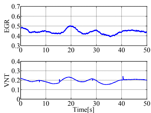
(d) MAP 目標値を変化させた 場合の入力
