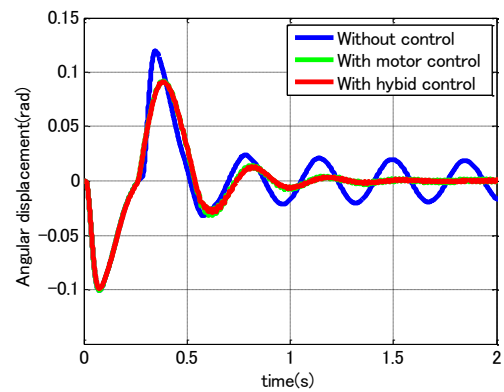
(b) 梁先端の角変位
