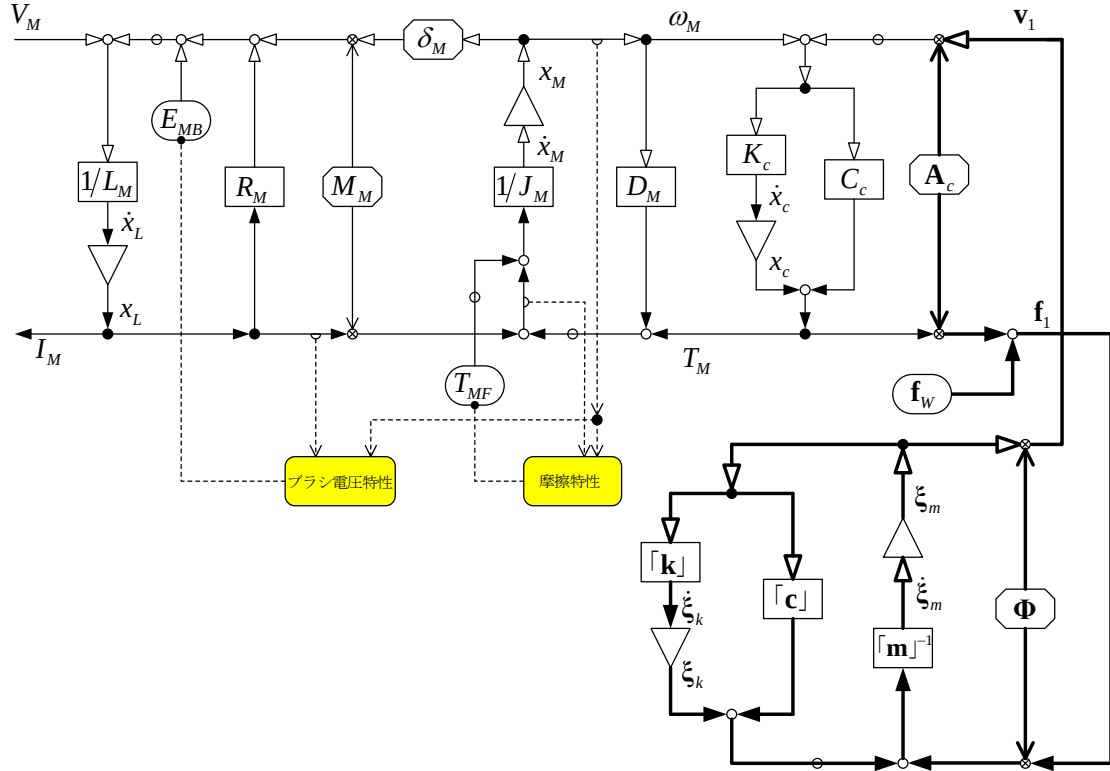
図 3.28 1 リンク機構の機能モデル
