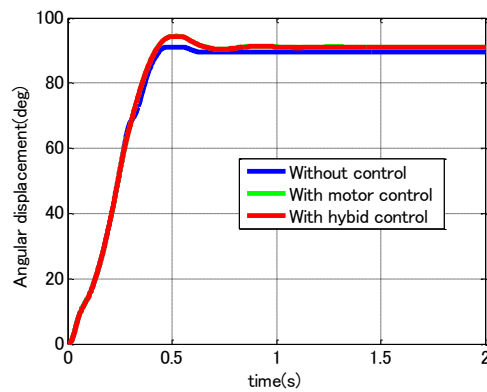
(a) モータの角変位
