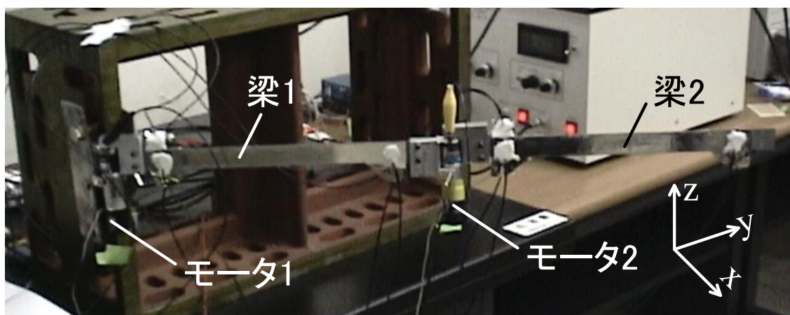
図 3.31 2 リンク機構の構成
