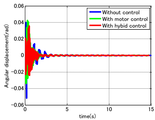
(d) 梁 2 先端の角変位
