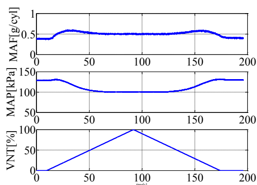
(b) VNT を変化させた場合 (EGR:28.5%)
