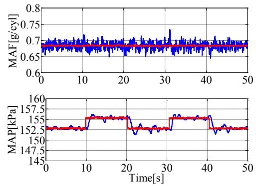
(d) MAP 目標値を変化させた 場合の応答 (実験結果)
