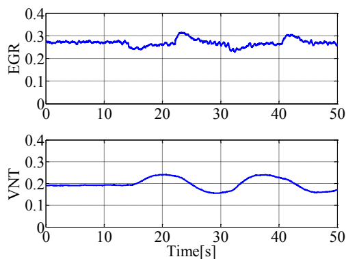
(c) MAF 目標値を変化させた 場合の入力
