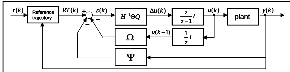
図 4.18 モデル予測制御ブロック線図
