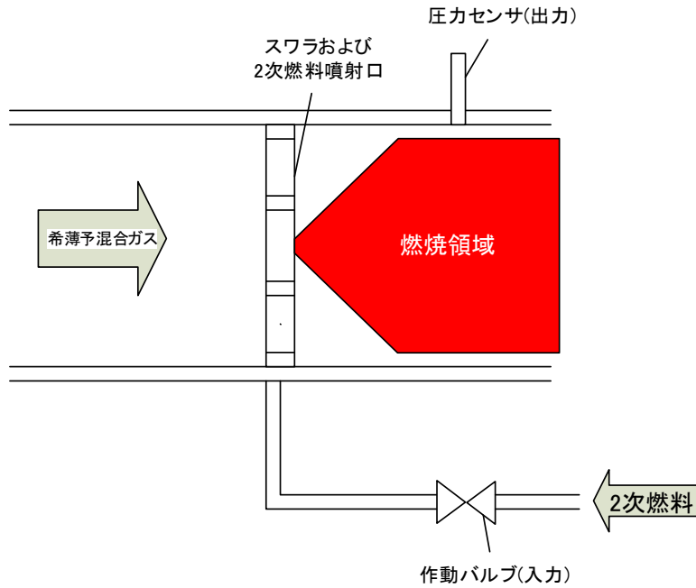
図 2.1 燃焼器概略図
