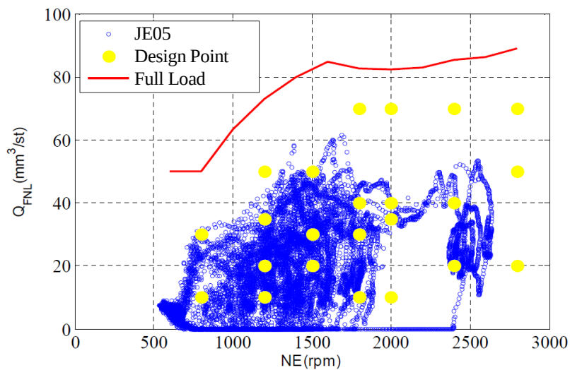
図 4.5 動作条件(設計点)
