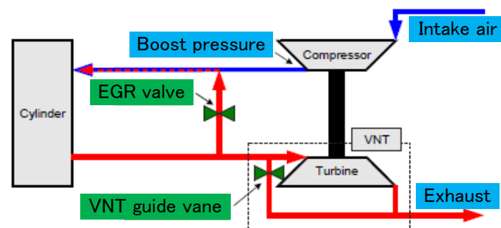
図 4.1 EGR/VNT 吸排気システム
