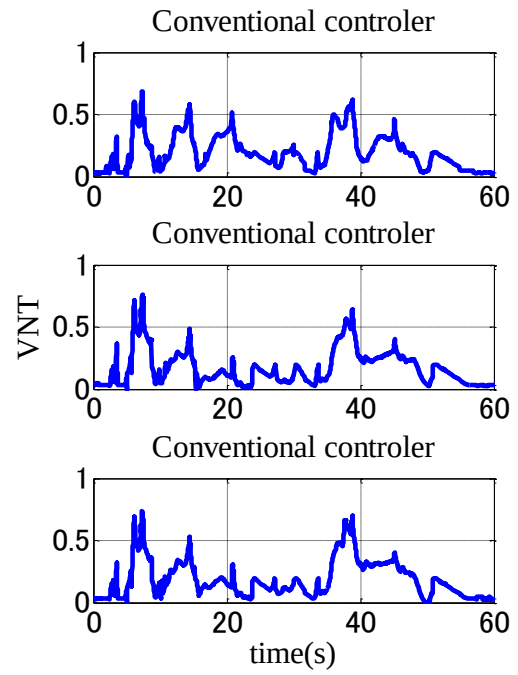
(b) VNT 指示開度
