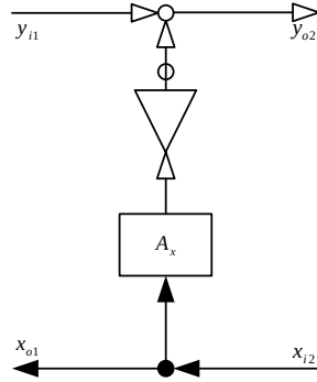
図 3.4 加算型-内包系の蓄積特性
