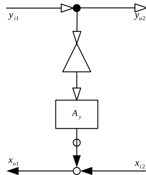
図 3.3 加算型-外延系の蓄積特性
