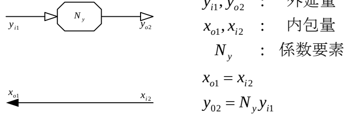
図 3.11 外延系の係数要素
