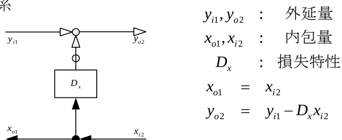
図 3.8 加算型-内包系の損失特性
