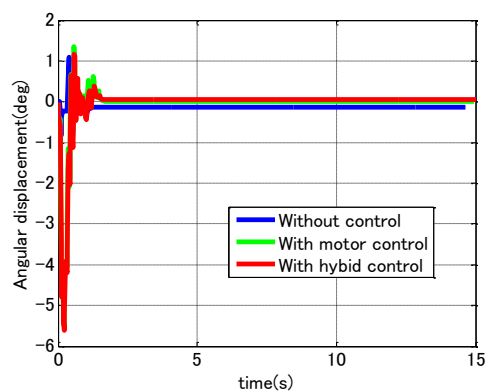
(b) モータ 2 の角変位
