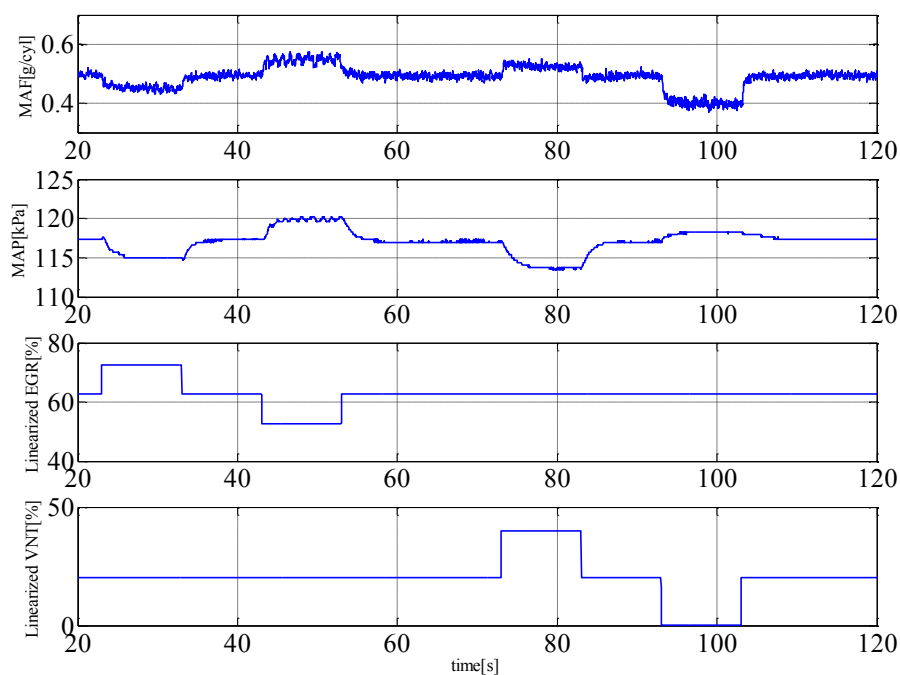
図 4.6 ステップ応答試験結果(1500rpm, 30mm 3 /st)
