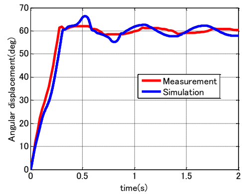
(b) モータ 1 の角度
