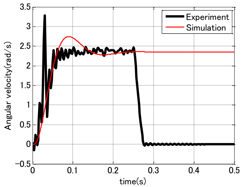
図 3.21 ステップ応答(5.0V)
