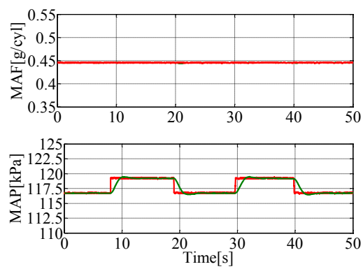
(b) MAP 目標値を変化させた 場合の応答 (シミュレーション結果)
