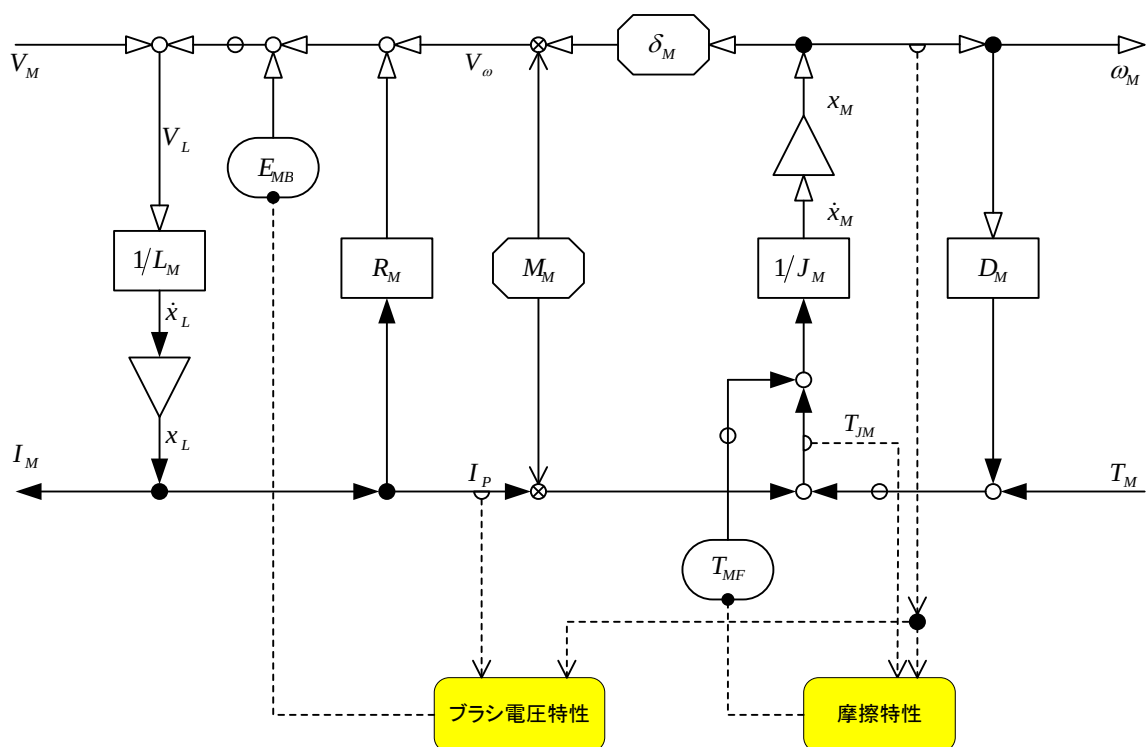
図 1.2 物理機能モデル(DC モータ)
