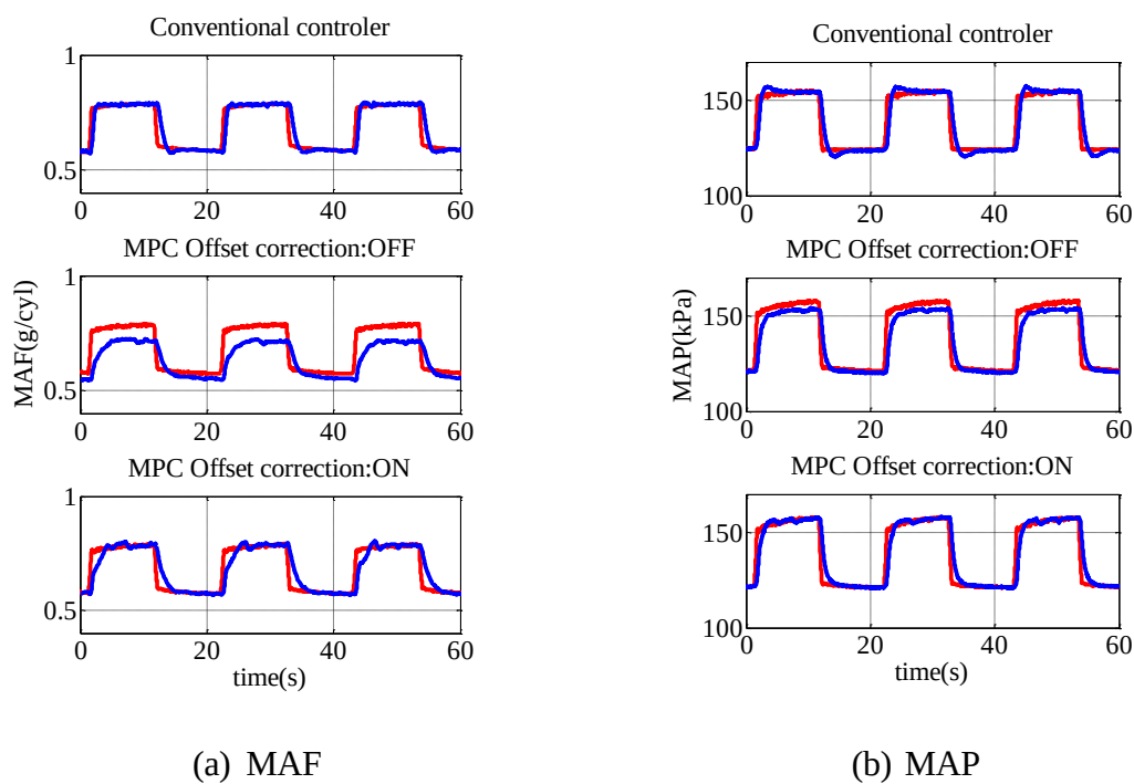
図 4.24 ステップ応答(2000rpm, 20 mm 3 /st → 40 mm 3 /st)
