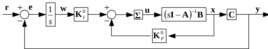
図 4.8 積分型最適サーボ系
