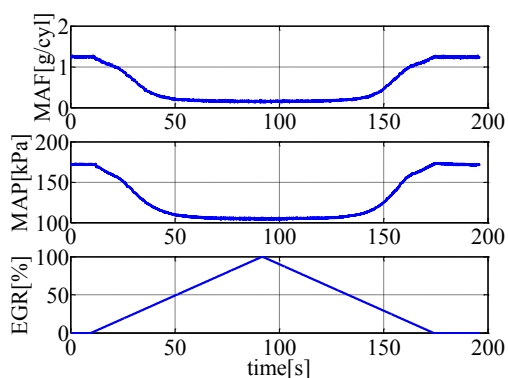
(a) EGR を変化させた場合(VNT:10.4%)
