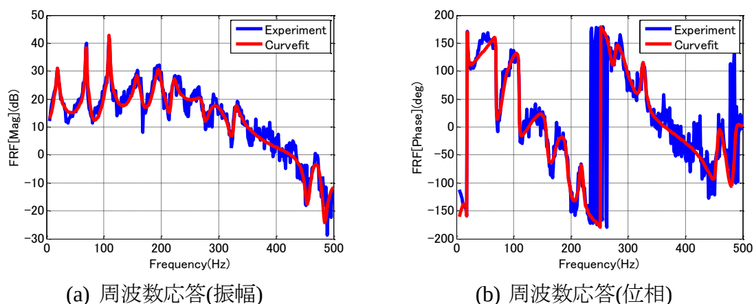
図 2.9 実験結果およびカーブフィット結果(当量比:0.39, シミュレーション用)
