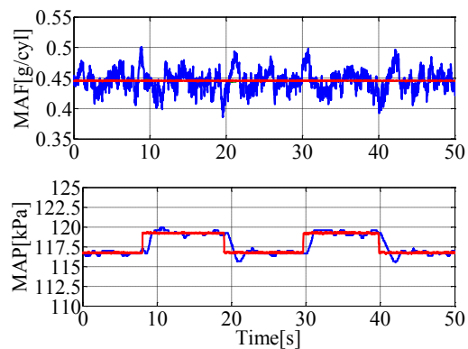
(d) MAF 目標値を変化させた 場合の応答 (実験結果)
