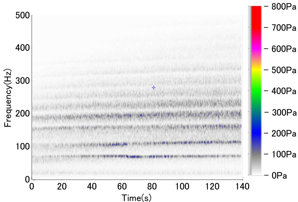
(b) 音圧のパワースペクトルマップ
