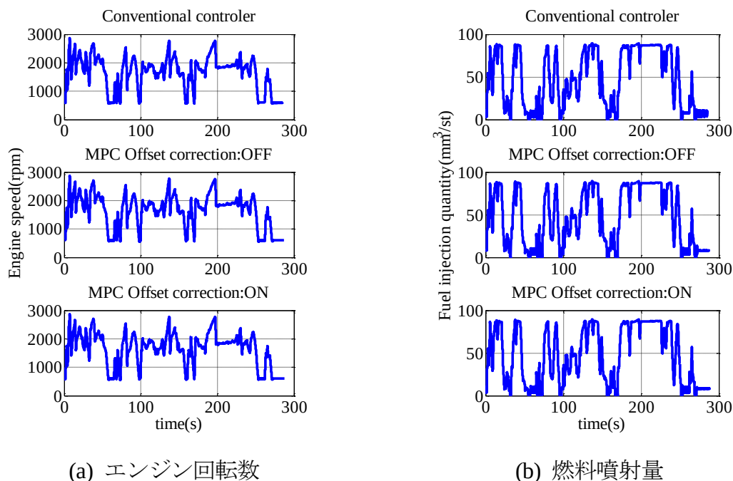
図 4.28 ETC モード
