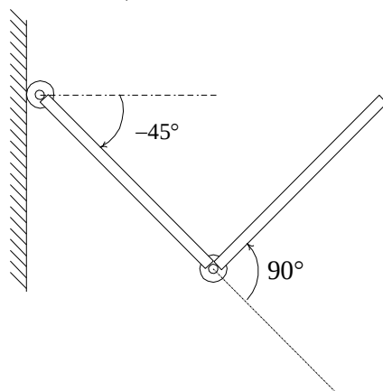
図 3.49 パターン3 ( \theta_1^* = -45^\circ, \theta_2^* = 90^\circ )
