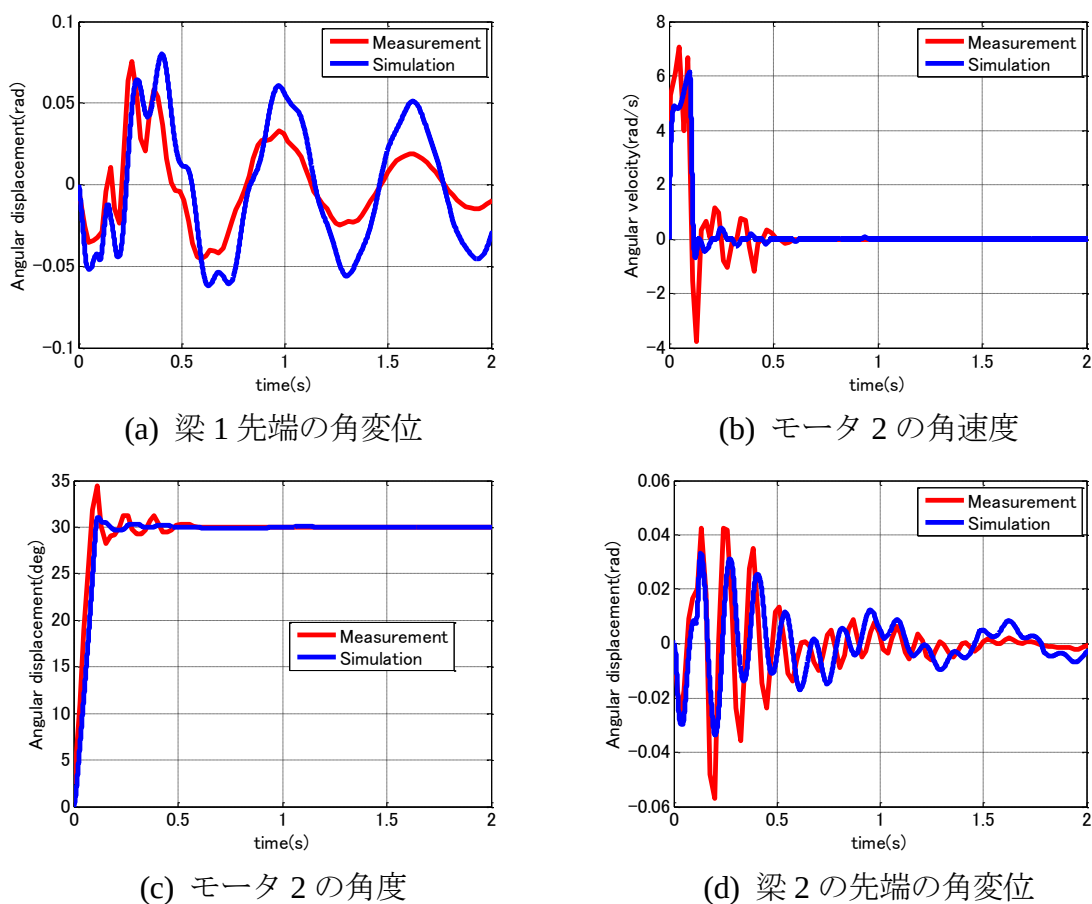
図 3.36 モータおよび梁の応答(パターン 1)
