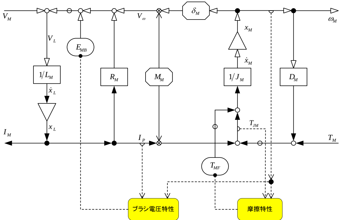
図 3.15 モータの回路
