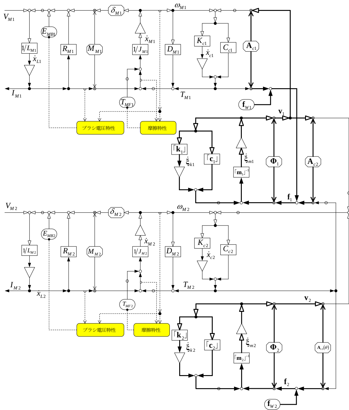
図 3.32 2 リンク機構の機能モデル
