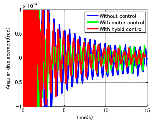
(f) 梁 2 先端の角変位(拡大)
