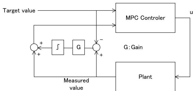
図 4.19 オフセット補正
