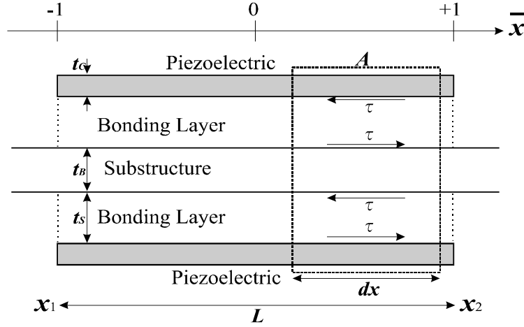
図 3.37 柔軟構造物と圧電フィルムの幾何学
