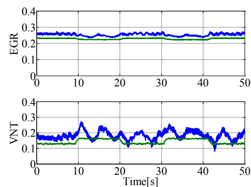
(e) MAF 目標値を変化させた 場合の入力
