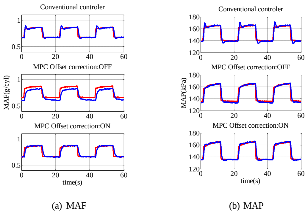
図 4.26 ステップ応答(2400rpm, 20 mm 3 /st → 40 mm 3 /st)
