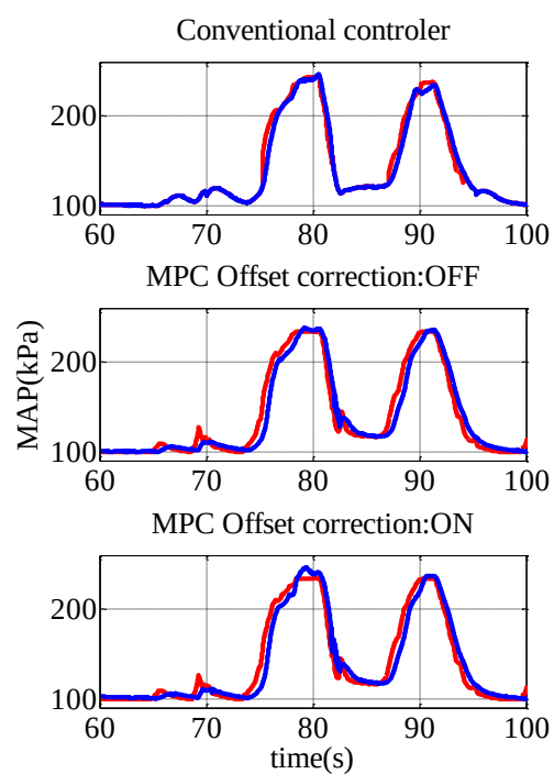
(d) MAP
