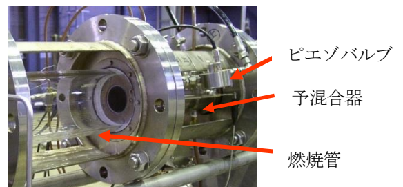
(b) 燃焼器(拡大)
