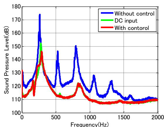
図 2.20 制御実験結果
