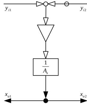
図 3.2 差分型-内包系の蓄積特性
