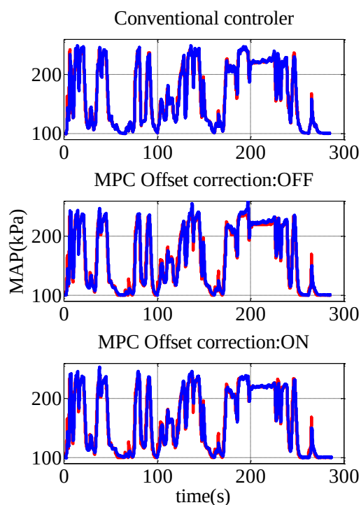
(d) MAP
