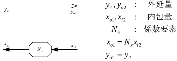
図 3.12 内包系の係数要素
