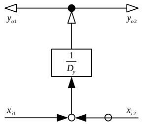
図 3.5 差分型-外延系の損失特性
