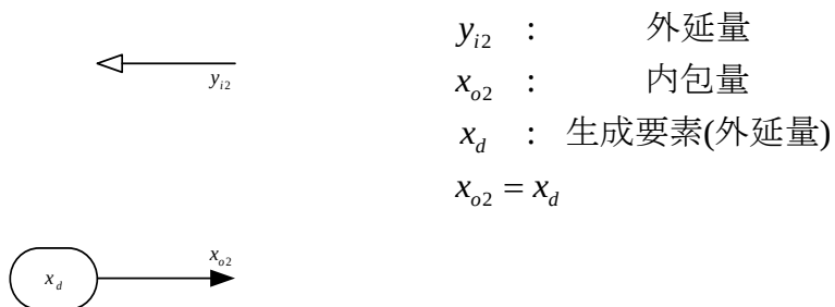
図 3.9 外延系の生成要素
