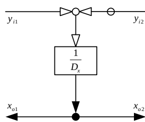
図 3.6 差分型-内包系の損失特性
