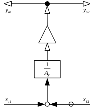
図 3.1 差分型-外延系の蓄積特性
