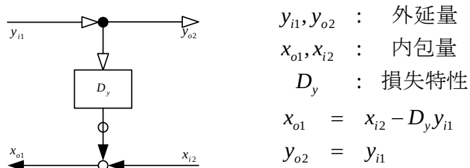
図 3.7 加算型-外延系の損失特性
