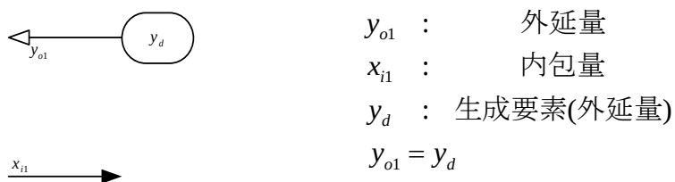
図 3.10 差分型-内包系の損失特性
