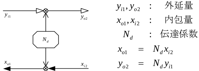
図 3.13 伝達係数要素
