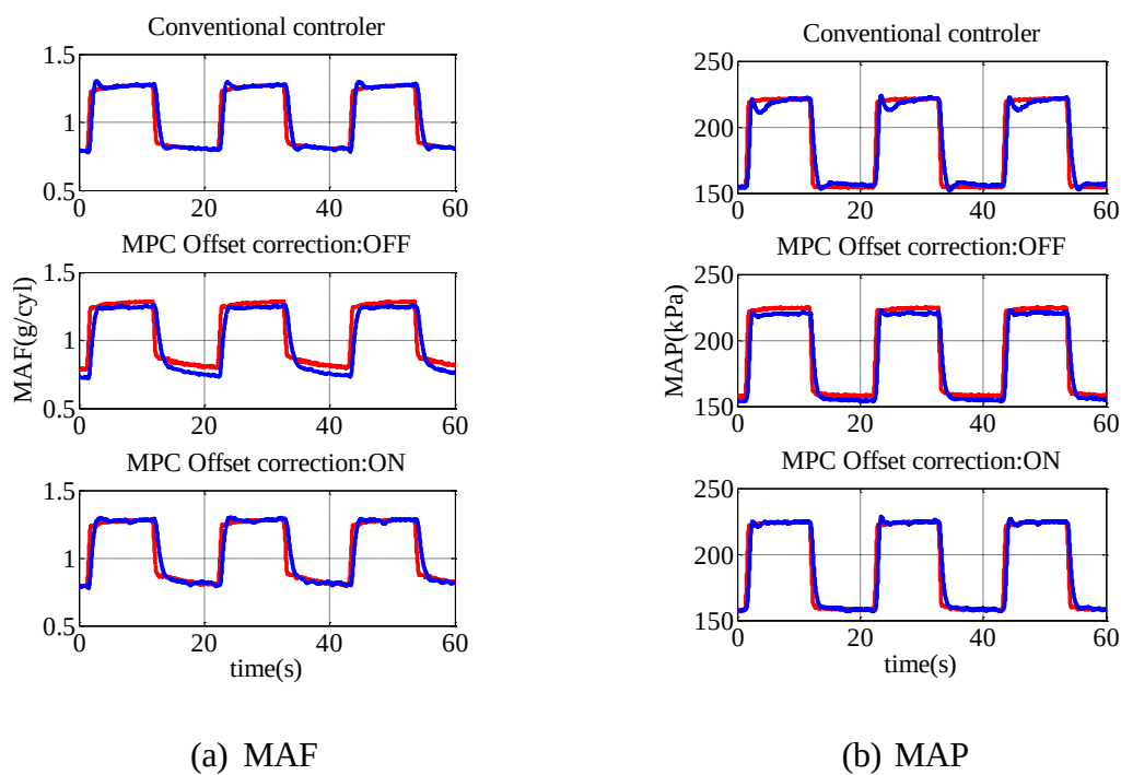
図 4.25 ステップ応答(2000rpm, 40 mm 3 /st → 80 mm 3 /st)
