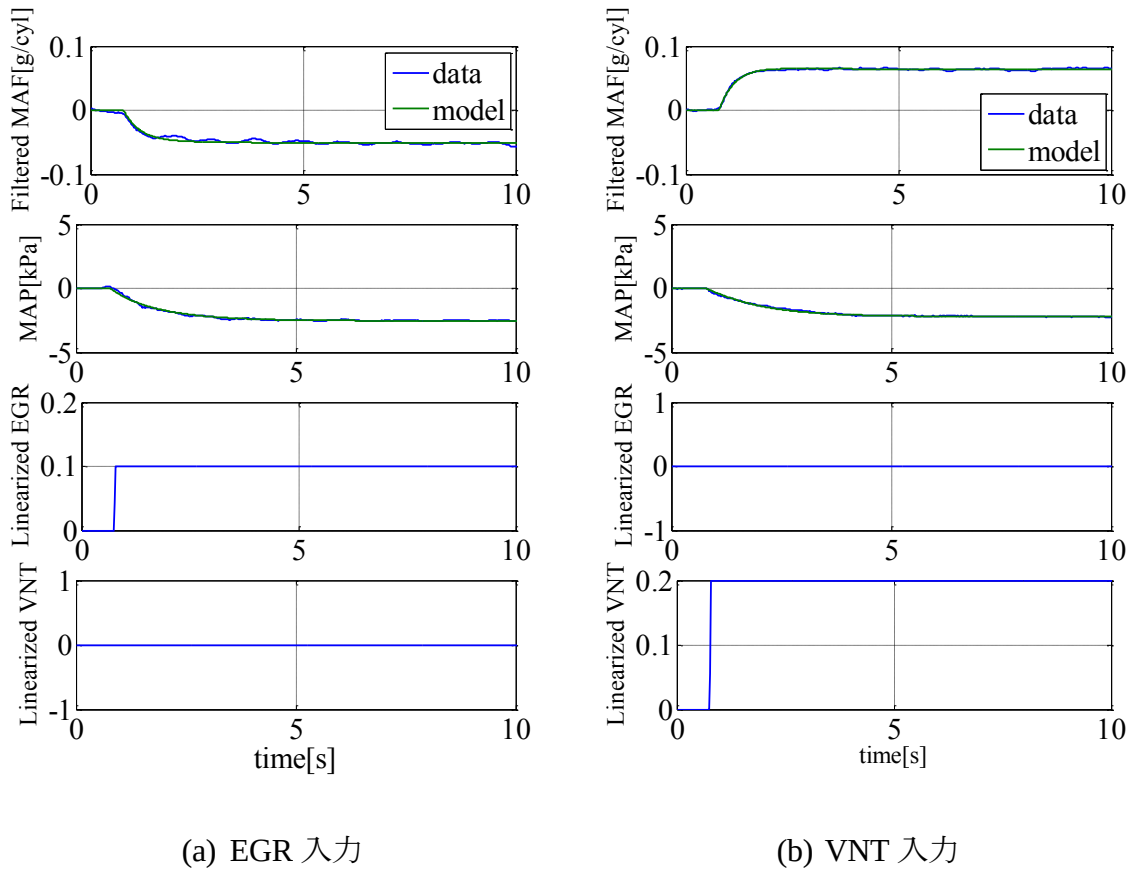
図 4.7 同定結果
