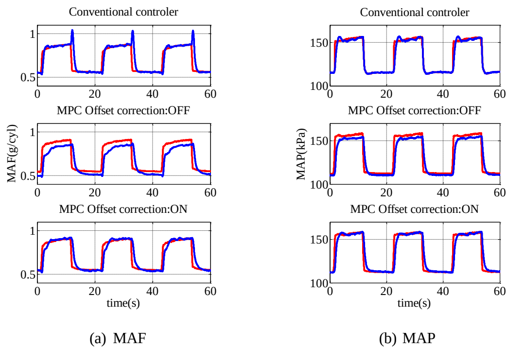
図 4.22 ステップ応答(1600rpm, 10 \text{ mm}^3/\text{st} \rightarrow 40 \text{ mm}^3/\text{st} )
