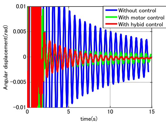
(e) 梁 1 先端の角変位(拡大)
