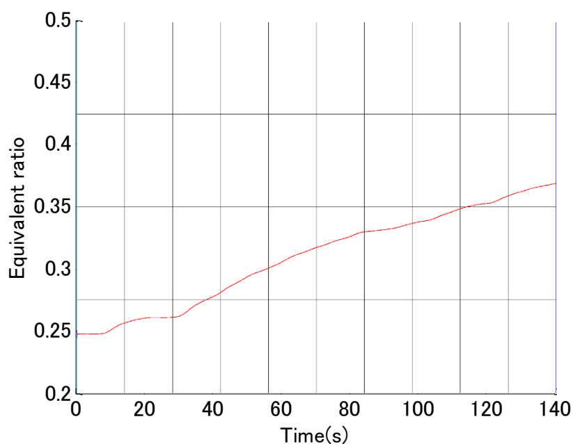
(a) 当量比
