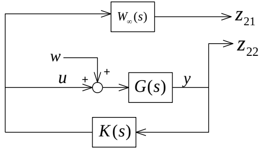
図 2.3 コントローラ設計のブロック線図
