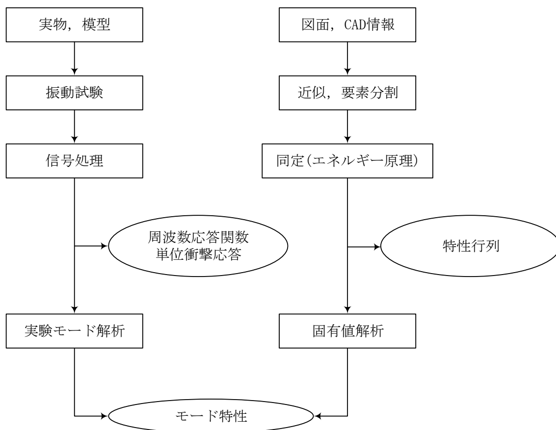
図 1.1 モード解析の流れ
