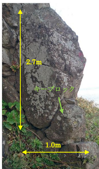
図 10 キーブロック拡大図
