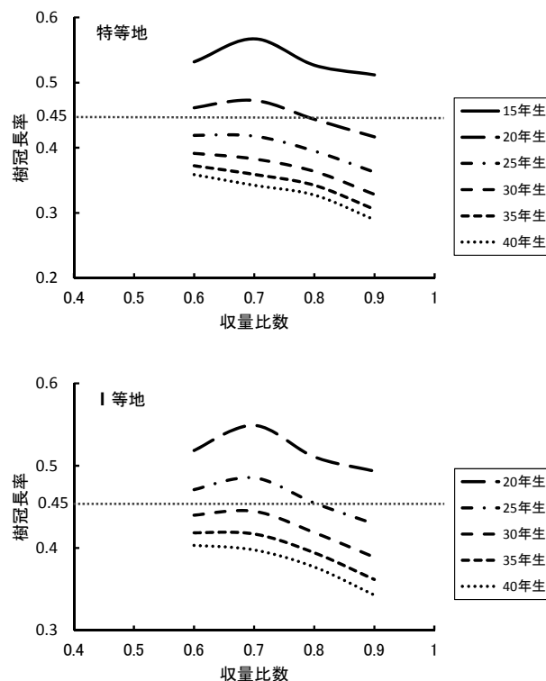
図4. 収量比数と樹冠長率の関係。
