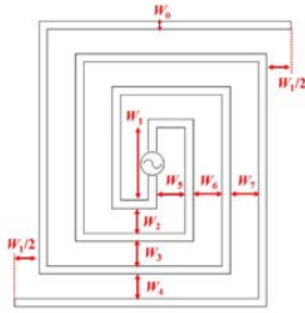
Fig. 1 Design parameters of PSA
