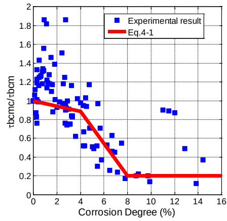
a. without stirrup
