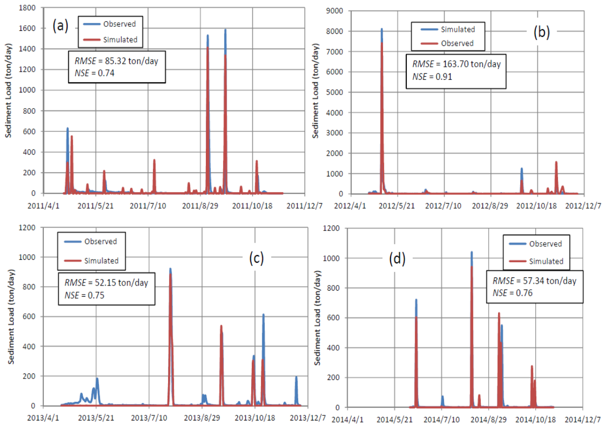
Fig. 4.4 Sediment load simulation at site R1 in 2011(a), 2012 (b), 2013 (c) & 2014 (d)
