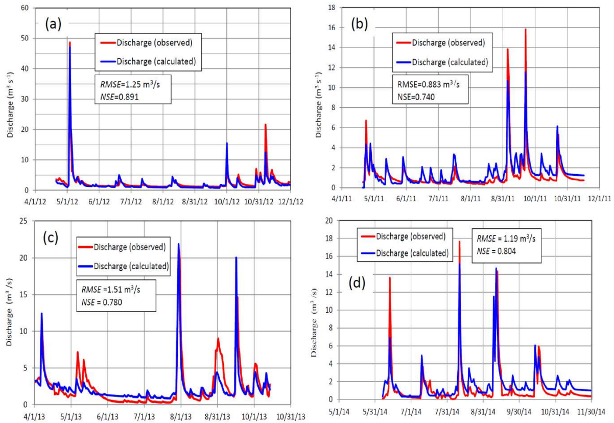
Fig. 3.3 Discharge simulation at site R1 (a) Calibration 2012 (b) validation 2011(c) validation 2013 (d) validation 2014.
