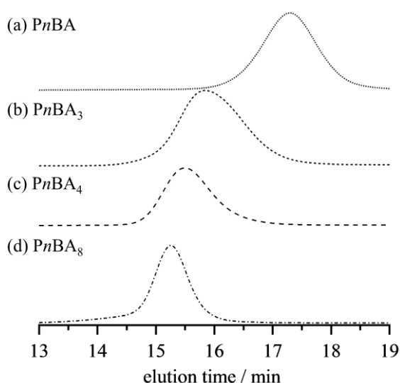
Figure 5-1. SEC traces (a) linear Pn BA, (b) Pn BA 3 , (c) Pn BA 4 , and (d) Pn BA 8 (eluent, THF; flow rate, 1.0 mL min -1 ).
