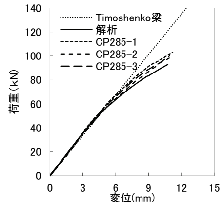
図-18 CP285荷重-変位関係
