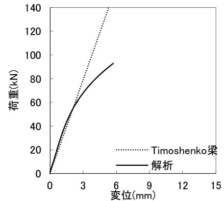
図-17 CP285せん断変形成分
