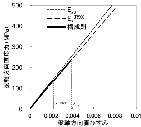
図-9 CP285の圧縮側応力-ひずみ挙動
