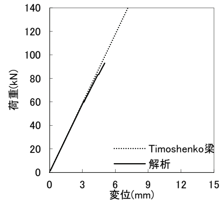
図-16 CP285曲げ変形成分
