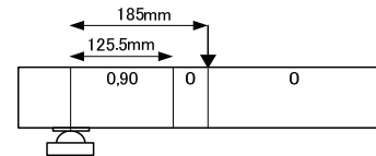
図-24 CP185 の破壊荷重時の上フランジ隅角部の健全層
