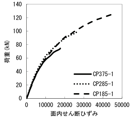
図5 荷重一面内せん断ひずみ関係
