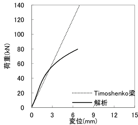
図-14 CP375のせん断変形成分
