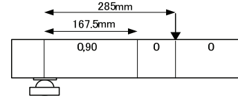
図-23 CP285 の破壊荷重時の上フランジ隅角部の健全層
