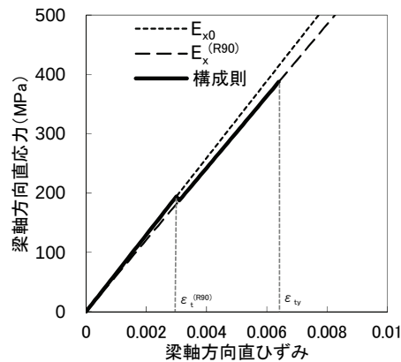
図-10 CP285の引張側応力-ひずみ挙動
