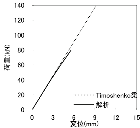
図-13 CP375の曲げ変形成分
