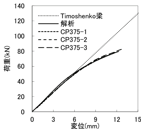
図-15 CP375の荷重-変位関係
