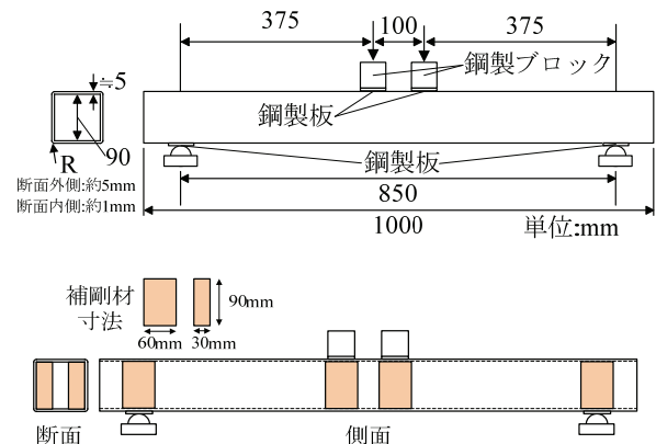
図-1 供試体寸法と载荷条件 (CP375)
