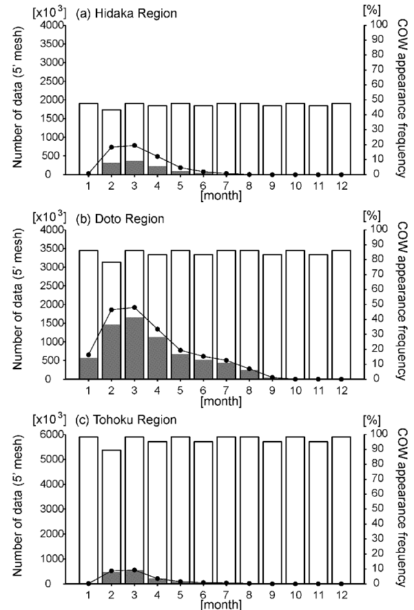
図5：沿岸親潮水の月別出現頻度(折線)。(a)はHidaka Region, (b)はDoto Region, (c)はTohoku Region. 白色棒グラフが各領域内でのプロファイル数、灰色棒グラフが沿岸親潮水を含むプロファイル数を示す。
