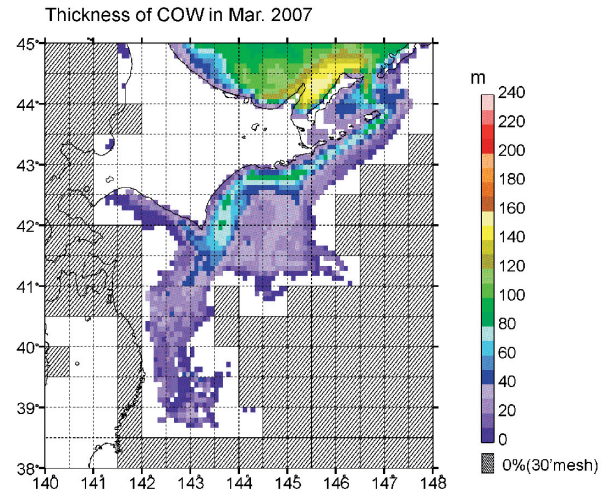
図7：2007年3月における沿岸親潮水の平均層厚。
