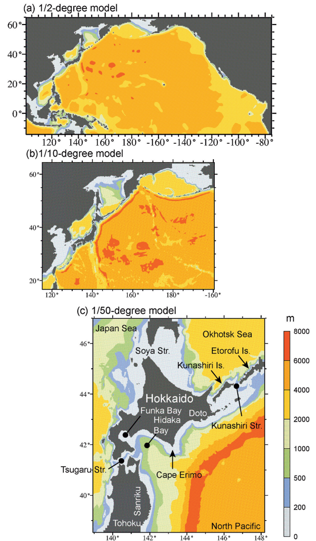
図 1: 海洋モデルの計算領域。 (a) は 1/2^\circ モデル, (b) は 1/10^\circ モデル, (c) は 1/50^\circ モデル
