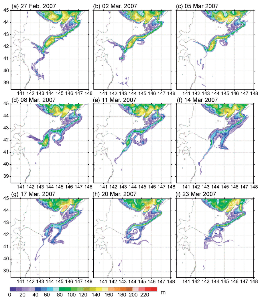
図8：2007年2月27日～3月24日における沿岸親潮水の層厚のスナップショット Figure 8 : Snapshots of thickness of the Coastal Oyashio Water from 27 February 2007 to 24 March 2007 in an interval of 3 days.
