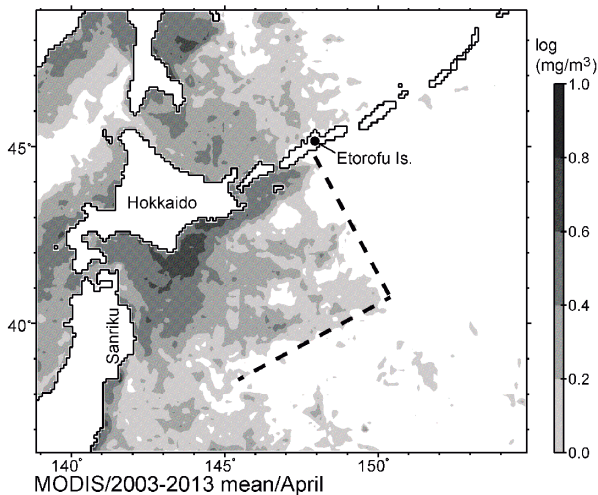
図9：MODIS Aquaによる2003年～2013年4月における11年平均海面クロロフィル濃度
