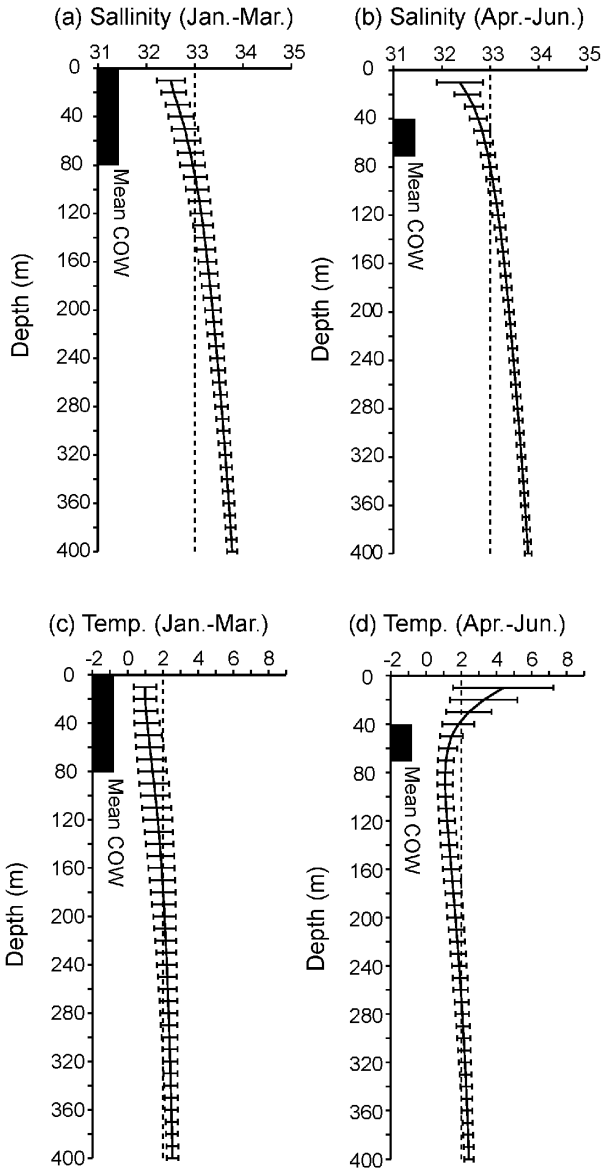
図6：Doto Regionにおいて沿岸親潮水を含む塩分（上段）および水温（下段）プロファイル（下段）の期間別平均。 (a)と(c)が1～3月平均、(b)と(d)が4～6月平均。平均プロファイルから検出される沿岸親潮水の深度範囲は黒領域で表示。
