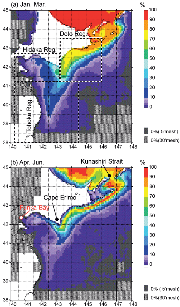
図2：沿岸親潮水の出現頻度。(a)は1～3月、(b)は4～6月。0%領域は黒色領域(5分メッシュ)と斜線領域(30分メッシュ)で表示。点線で囲まれた領域は、Hidaka Region(北西側の領域)、Doto Region(北東側の領域)、Tohoku Region(南側の領域)と参照される。
